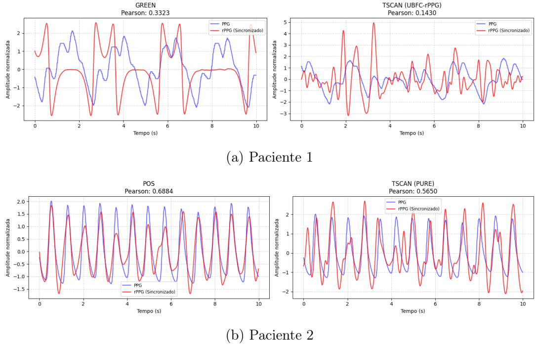
Figura 14: Sinais de rPPG dos métodos que obtiveram o maior coeficiente de correlação de Pearson com o sinal de PPG de referência em cada paciente, considerando o alinhamento temporal realizado por meio de correlação cruzada.
