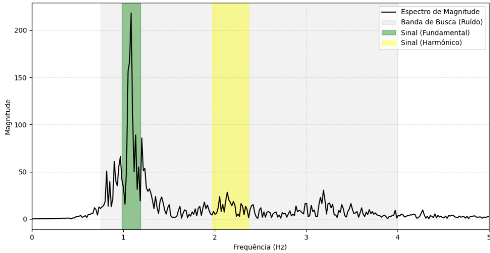
Figura 10: Exemplo da definição da relação sinal-ruído
