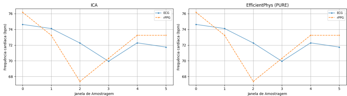
Figura 22: Estimativas de frequência cardíaca por janela dos sinais que resultaram no menor erro médio absoluto.
