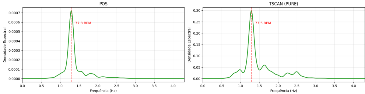
Figura 16: Espectros de potência de dois dos sinais de rPPG cujas estimativas de frequência cardíaca resultaram no menor erro absoluto médio em relação às estimativas obtidas por meio do ECG
