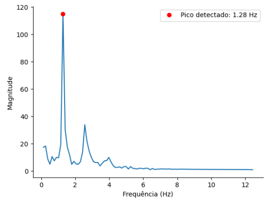
(b) Detecção do pico do espectro de frequência do sinal de BVP
