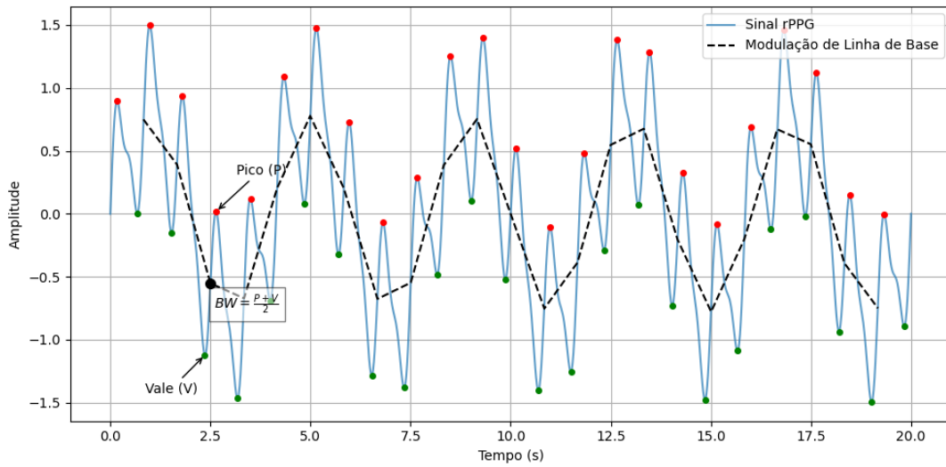
Figura 6: Extração da modulação de linha de base no sinal de rPPG causada pela respiração
