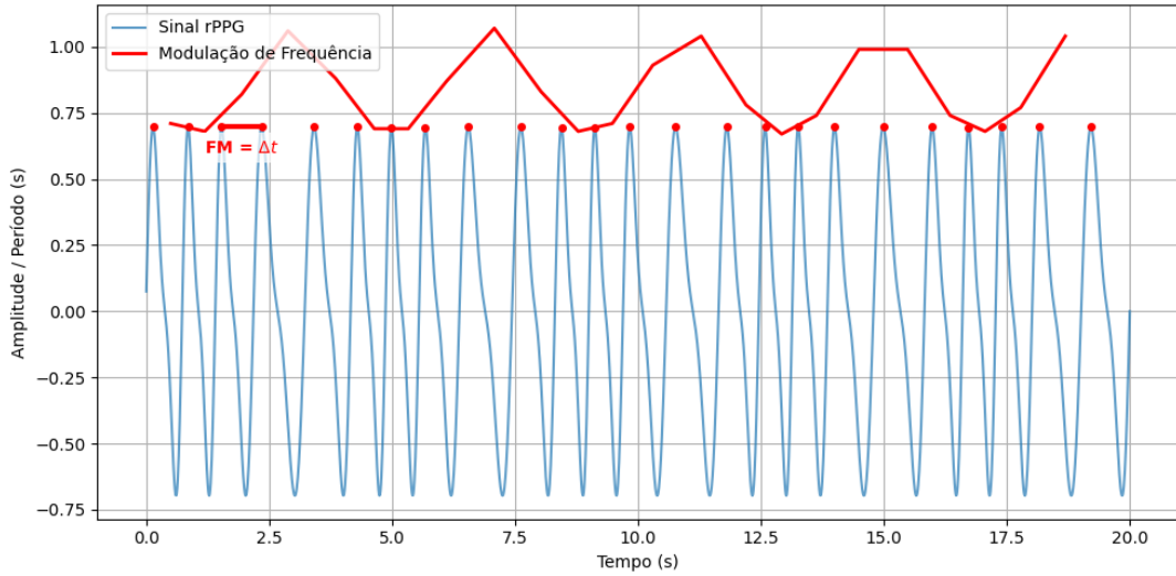
Figura 8: Extração da modulação de frequência do sinal de rPPG causada pela respiração Fonte: autoria própria
