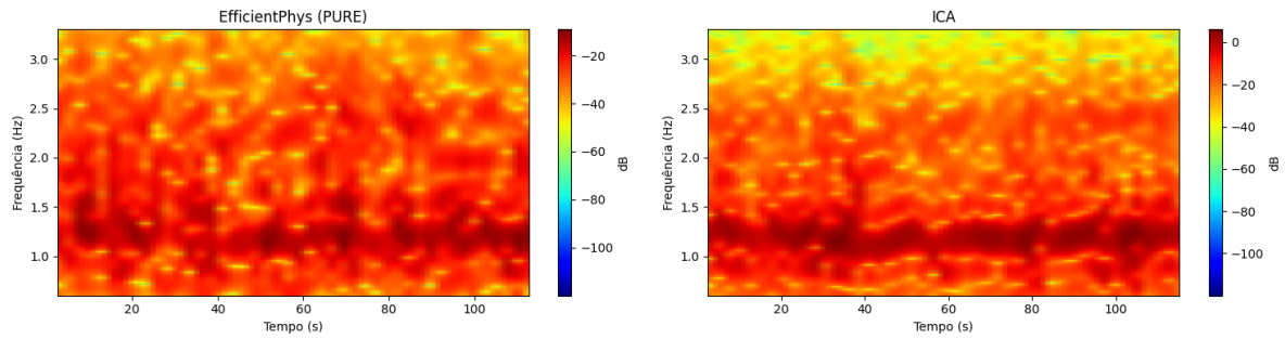
Figura 20: Espectrogramas dos sinais cujas estimativas de frequência cardíaca resultaram no menor erro médio absoluto.
