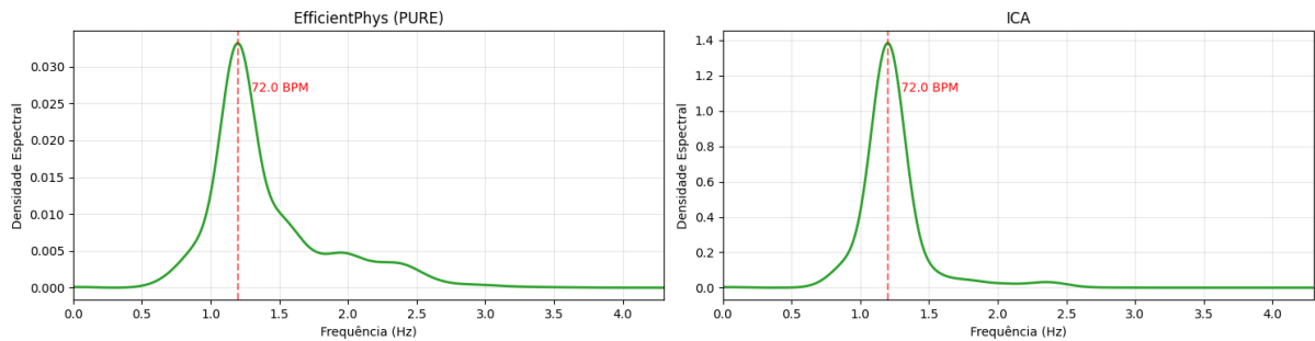
Figura 21: Espectros de potência dos sinais cujas estimativas de frequência cardíaca resultaram no menor erro médio absoluto.
