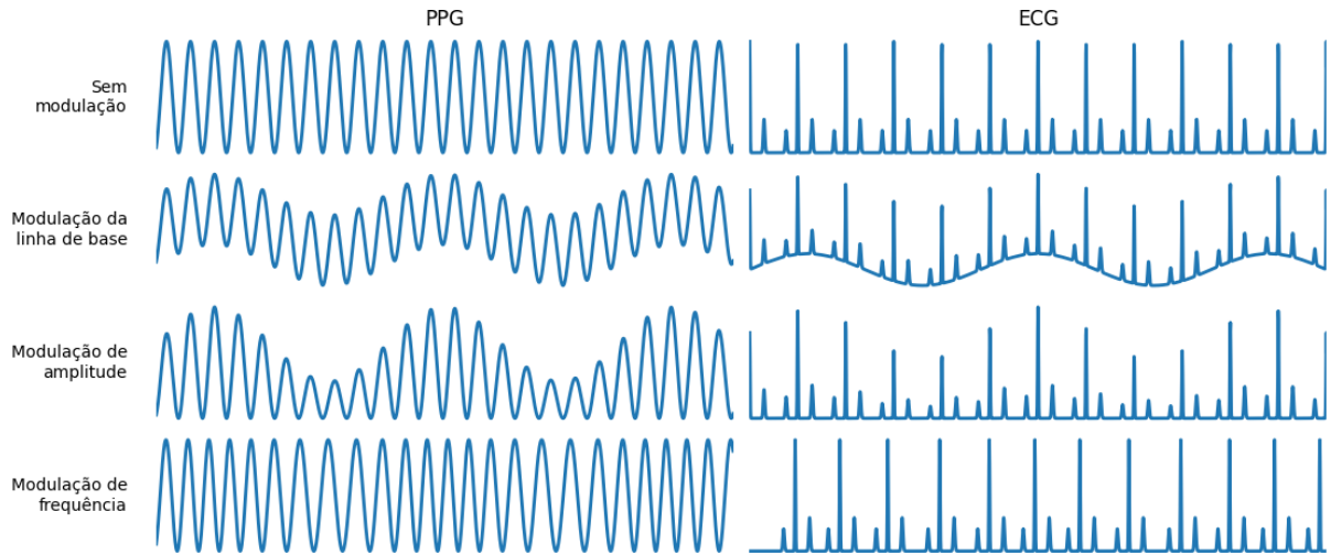
Figura 4: Tipos de modulação dos sinais de ECG e PPG causados pela respiração Fonte: Adaptado de Charlton et al. (2016)
