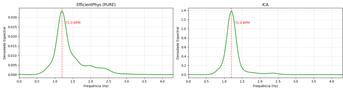
Figura 15: Espectros de potência dos sinais cujas estimativas de frequência cardíaca resultaram no menor erro médio absoluto.
