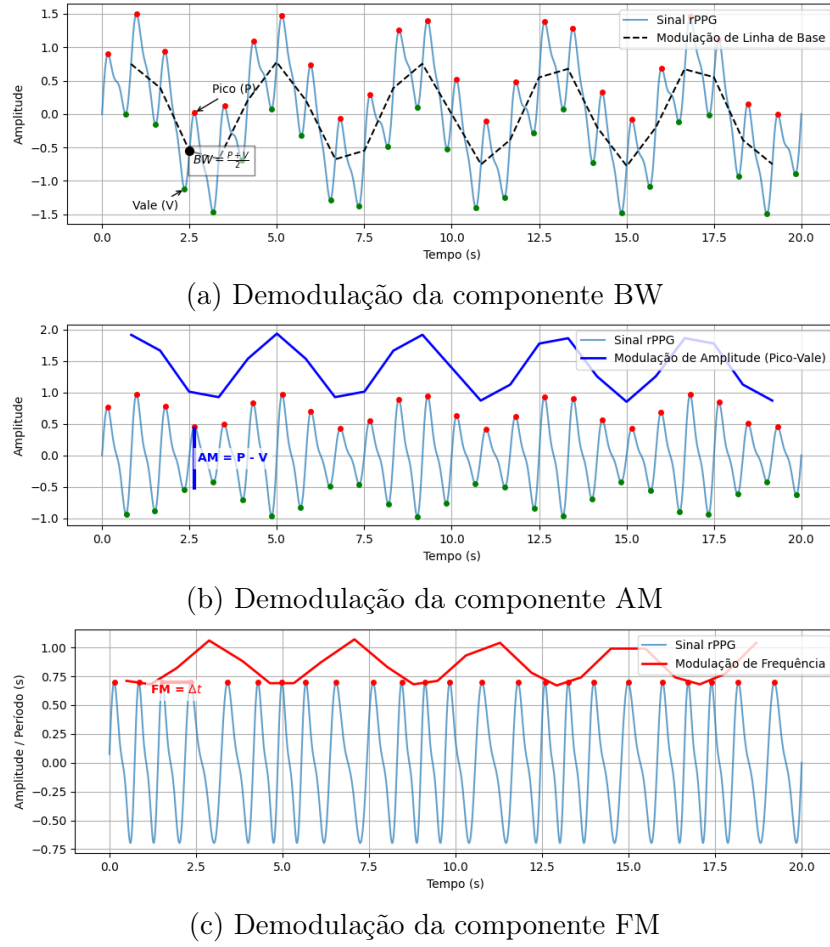
Figura 7: Estratégias de extração de cada modulação gerada pela respiração a partir do sinal de rPPG
