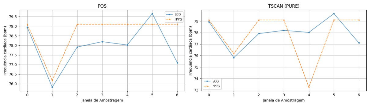
Figura 12: Estimativas de frequência cardíaca por janela obtidas por meio de dois dos métodos de rPPG que resultaram no menor erro absoluto médio em relação às estimativas obtidas por meio do ECG
