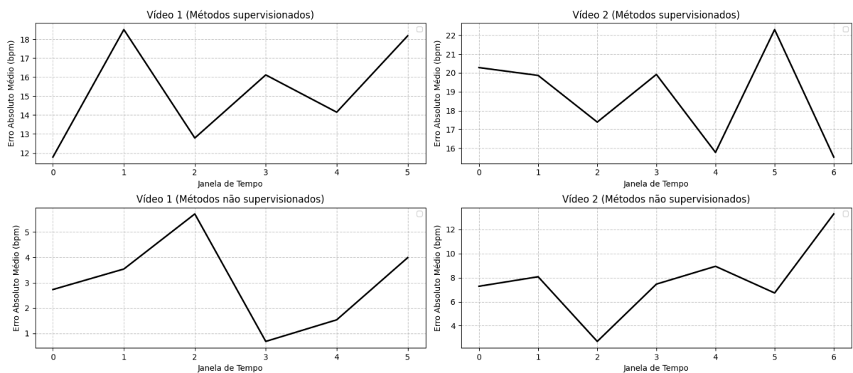
Figura 17: Erro absoluto médio por janela dos métodos supervisionados e não supervisionados de cada vídeo da coleta 2.
