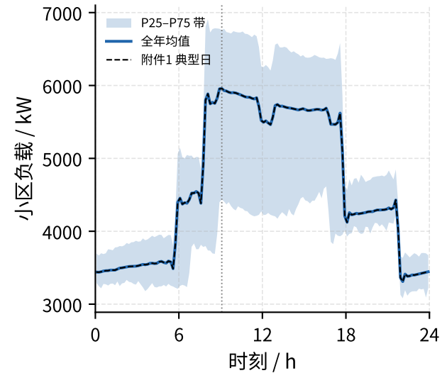
小区负载
