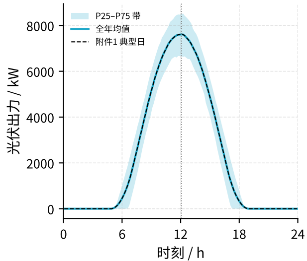
光伏出力
