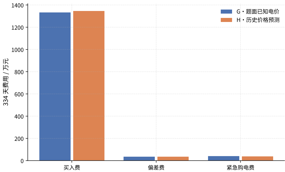
图 6 波动电价调整层在 G、H 两种信息条件下的费用分解
