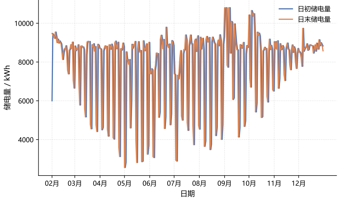
图 3 问题二实际储能电量及日末电量变化
