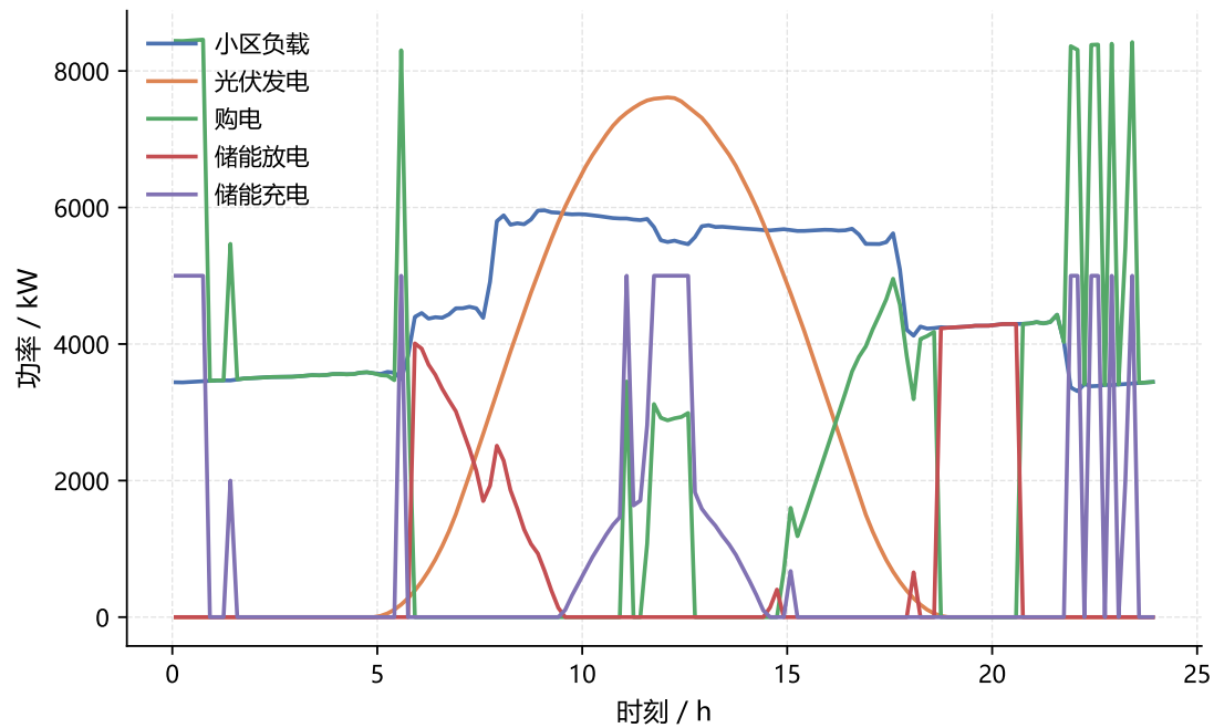
图 2 典型日购电、光伏与储能联合调度
