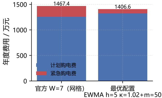
(d) 官方 vs 最优配置
