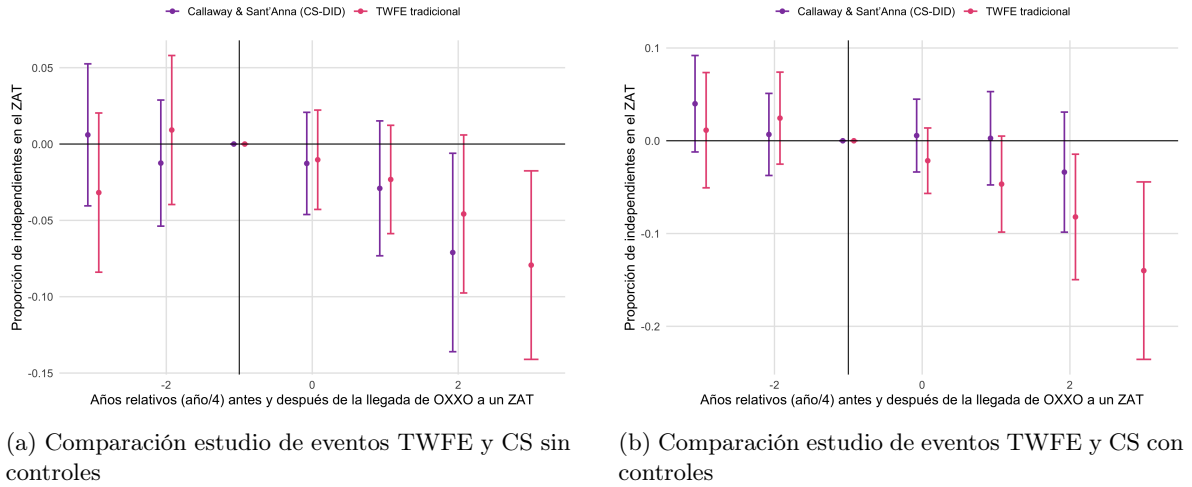
Figura 4: Comparación estudio de eventos TWFE y CS.
