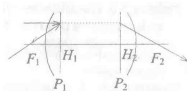
Рис. 5.1.1. Хід променів у товстій лінзі.
