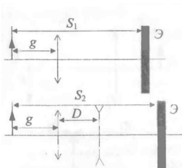
Рис. 5.1.4. Визначення фокусної відстані розсіювальної лінзи
