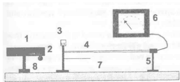
Рис. 5.6.3. Схема експериментальної установки.
