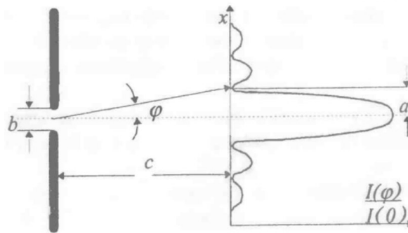
Рис. 5.6.1. Дифракція в паралельних променях.
