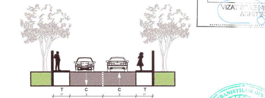
E - PROFIL STRADAL: Drum de servicii locale - 3 m T: Traseu; C: Cămin
