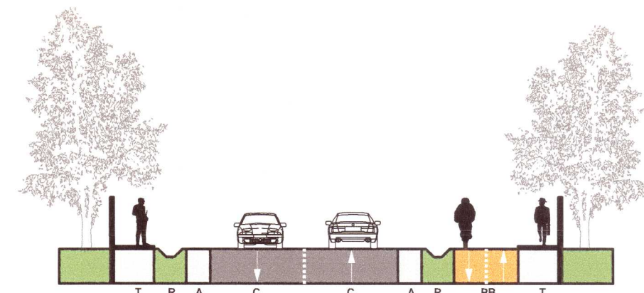
B - PROFIL STRADAL: Drum județean/comunal - 16,8 m (peste 13,90 m) T: Traseu; P: Pârâie de scolare; C: Cămin; A: Autostanție; R: Regimul inundațiilor
