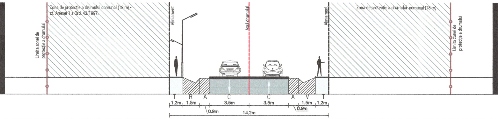
Profil stradal drum comunal - 14.2 m
