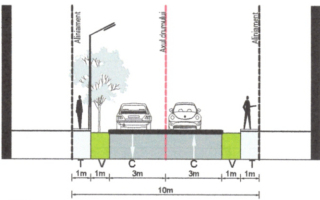
Profil străzi secundare și ulițe - 10 m
