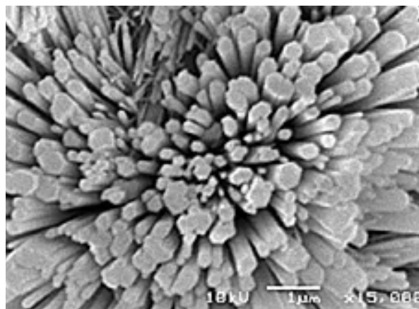
AQB RE-CRYSTALLIZED HA / SEM
