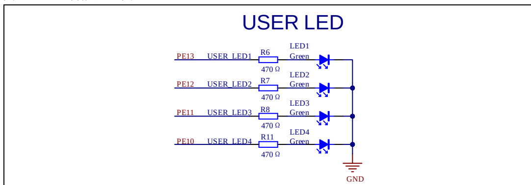
图3-3. LED功能原理图
