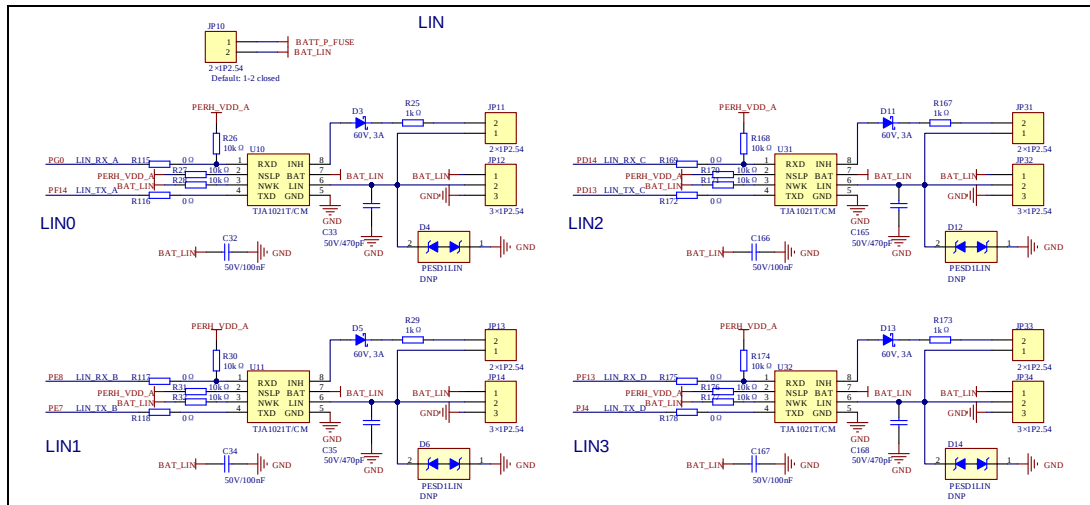
图3-8. LIN原理图
