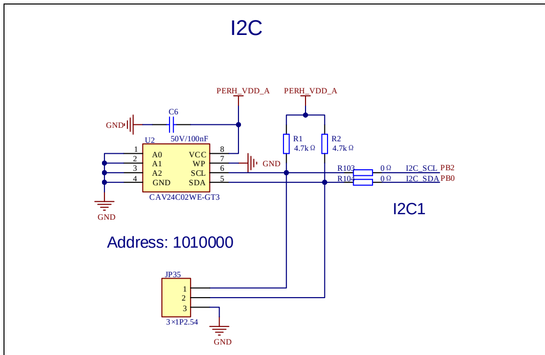
图3-9. I2C原理图
