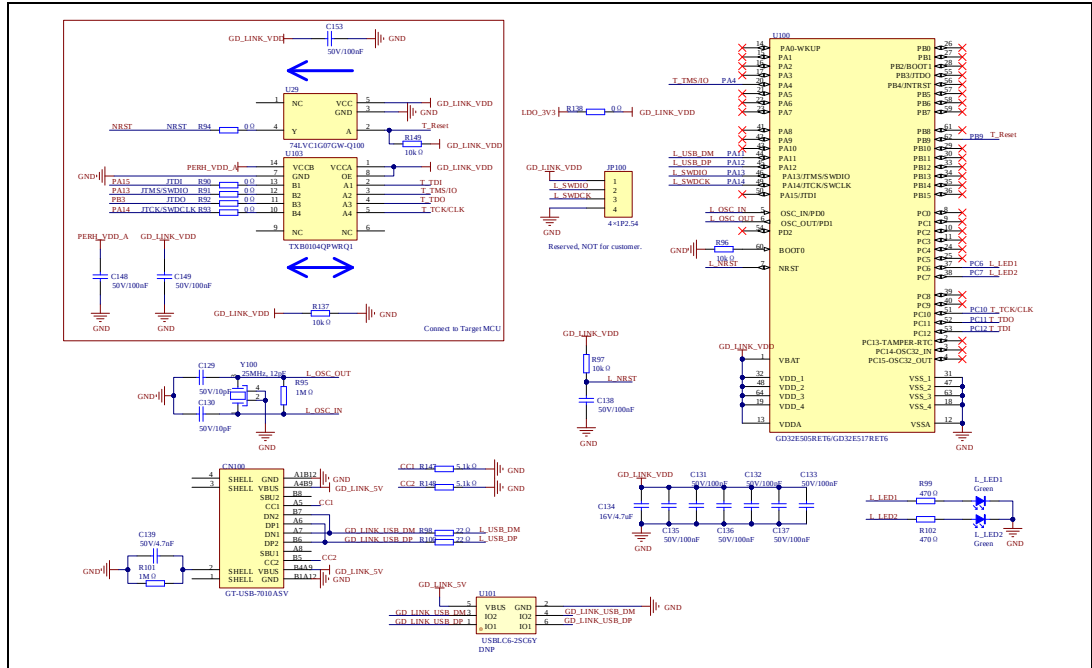
图3-15. GD-Link原理图
