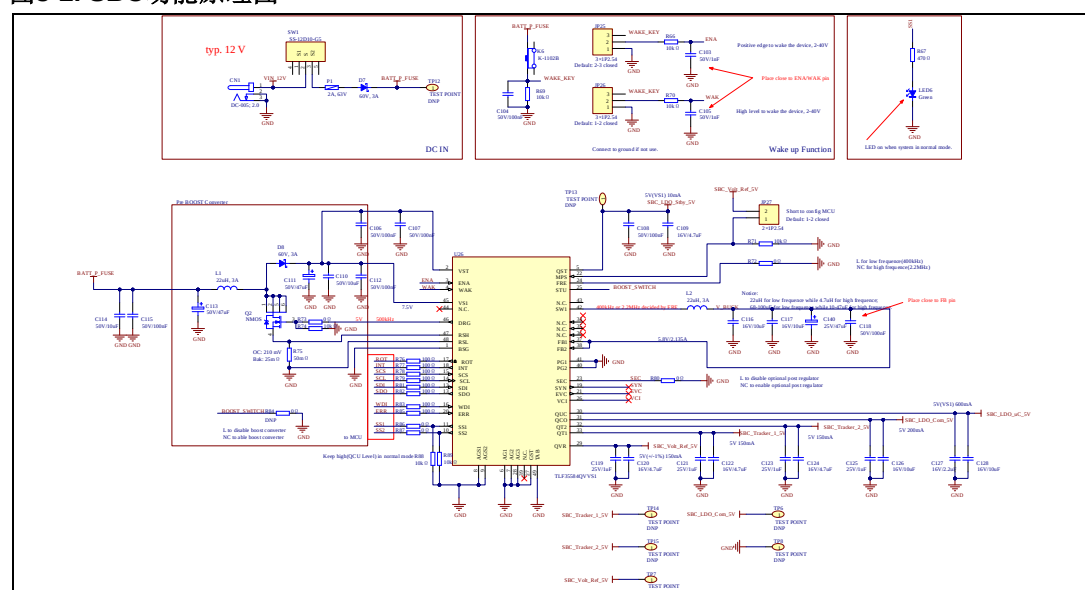
图3-2. SBC功能原理图
