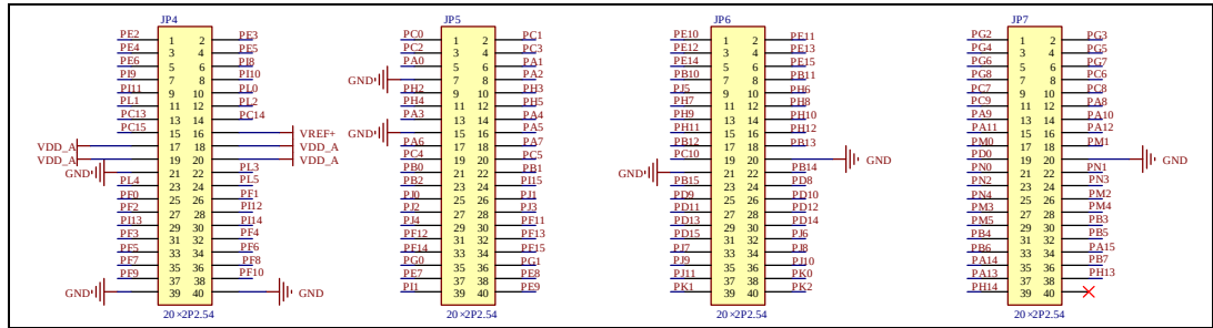
图3-14. Extension原理图
