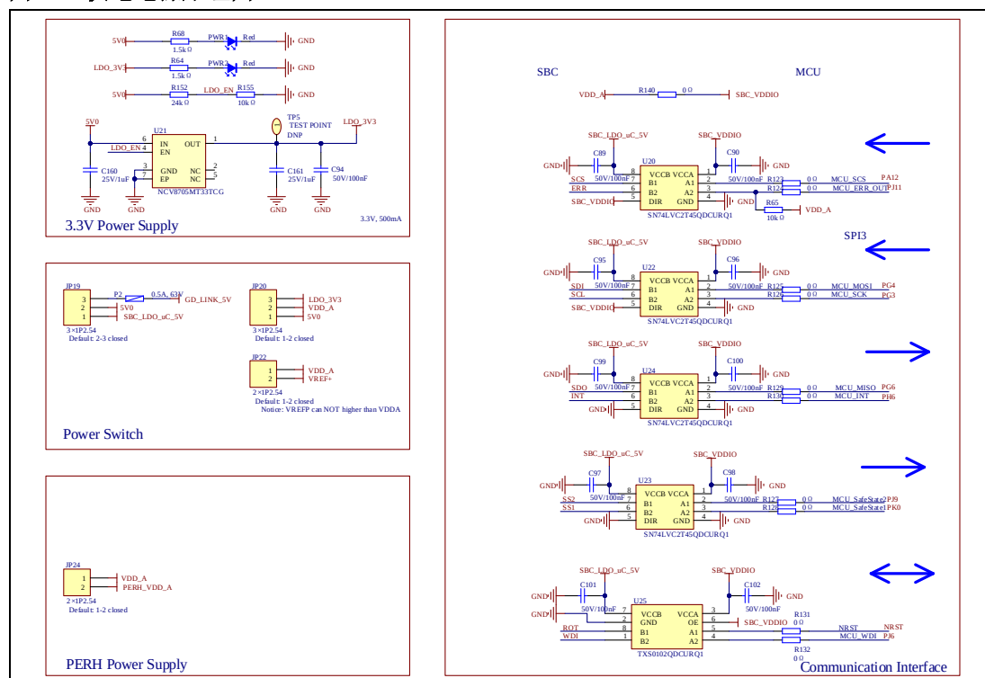
图3-1. 供电电源原理图
