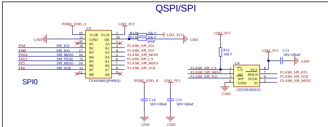
图3-12. SPI flash原理图
