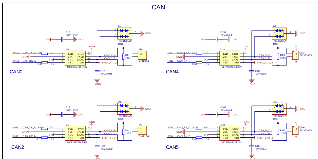
图3-7. CAN原理图
