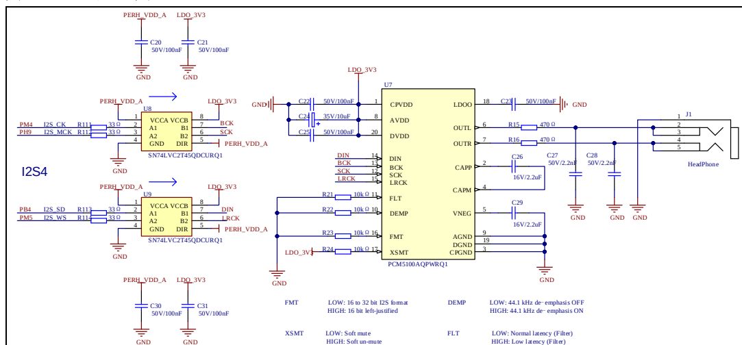
图3-10. I2S原理图
