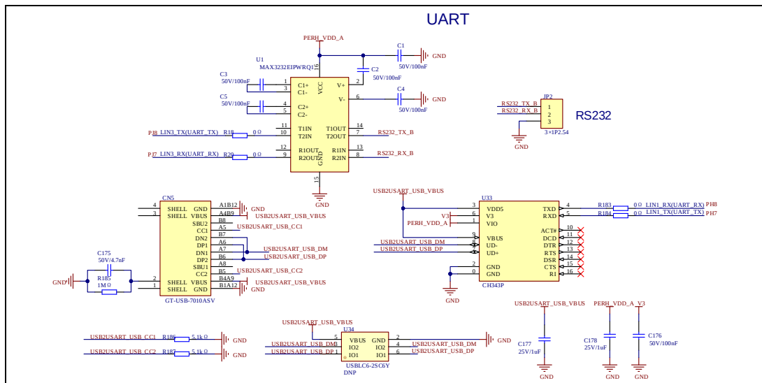
图3-13.UART原理图
