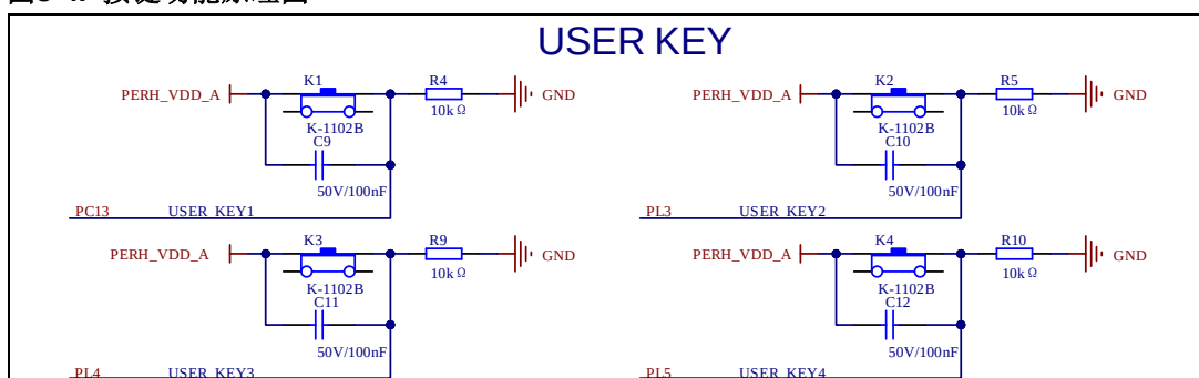
图3-4. 按键功能原理图
