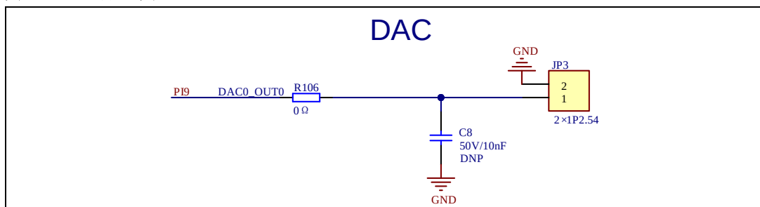
图3-6. DAC原理图
