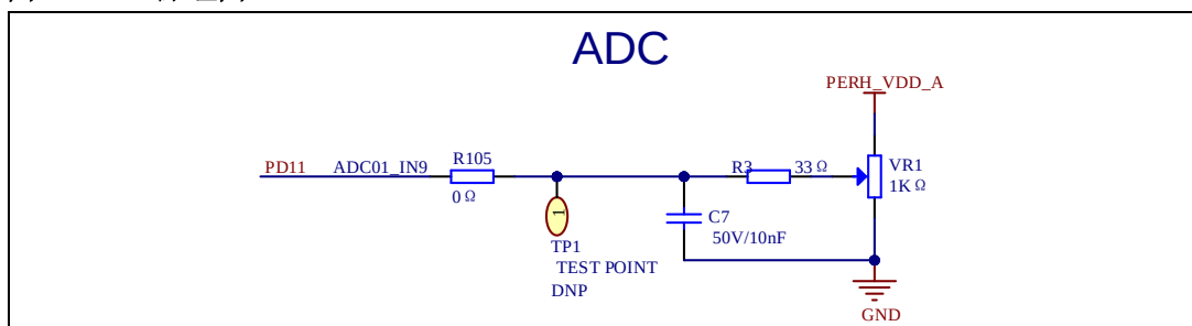
图3-5. ADC原理图
