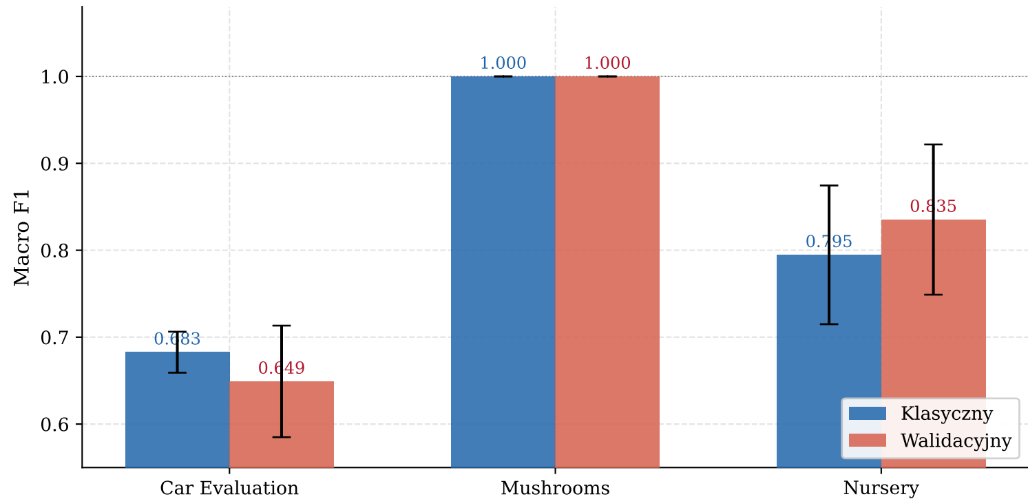
Macro F1 na zbiorze testowym — porównanie wariantów ( b = 30 , podział 60/20/20%, n = 5 podziałów, słupki błędów = \pm\sigma )
