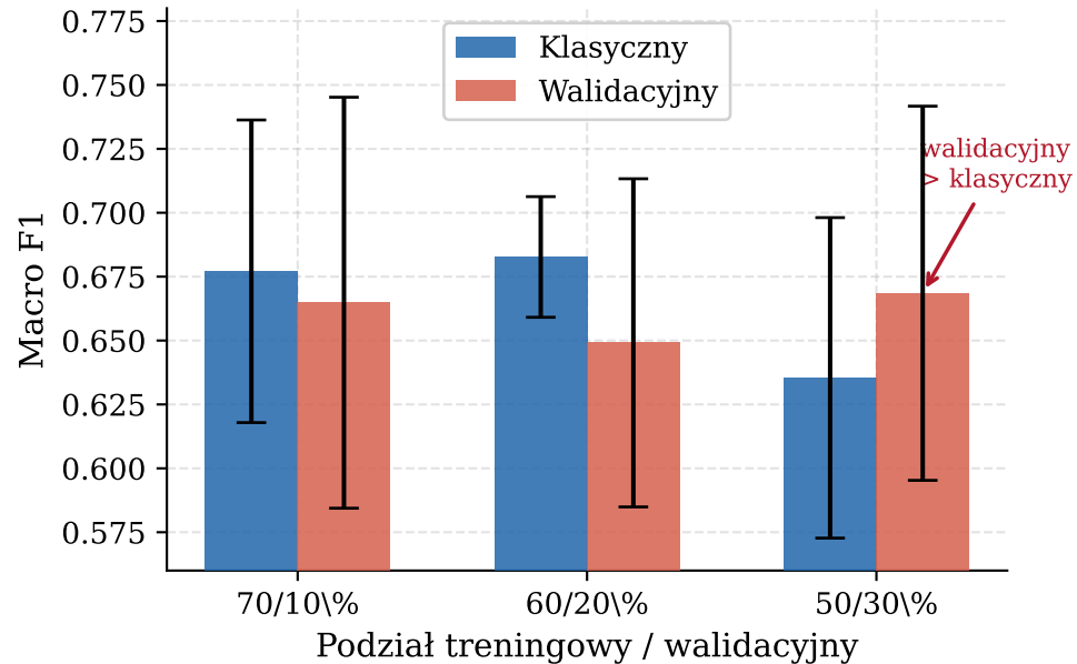
Macro F1
