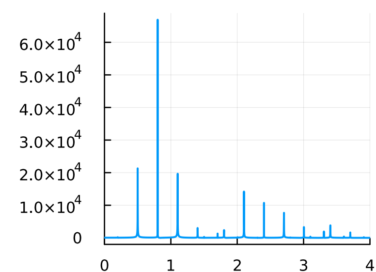
F=1.0, \omega=0.5
