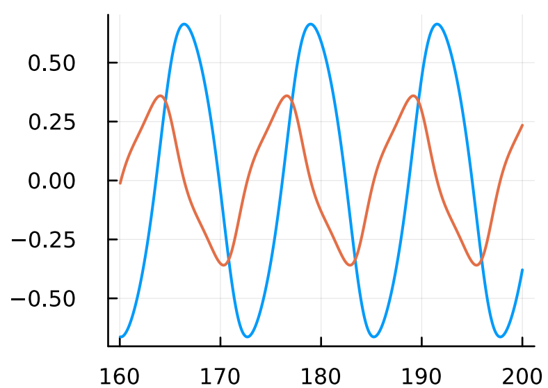
F=1.0, \omega=0.5
