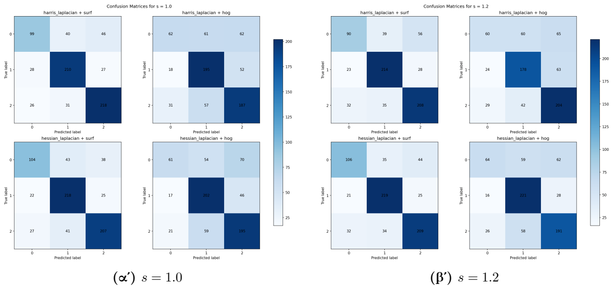
Σχήμα 47. Confusion matrices για s = 1.0 και s = 1.2 .
