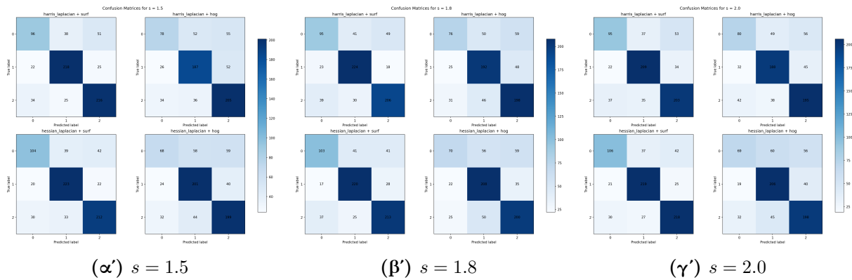
Σχήμα 48. Confusion matrices για s = 1.5 , s = 1.8 και s = 2.0 .
