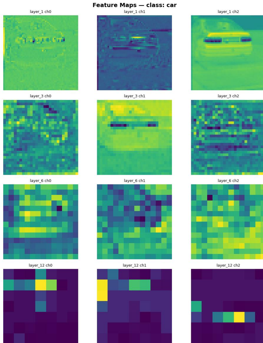
Σχήμα 50. Χάρτες ενεργοποίησης (3 κανάλια) για τα επίπεδα layer_1 , layer_3 , layer_6 , layer_12 για τη κλάση: car .
