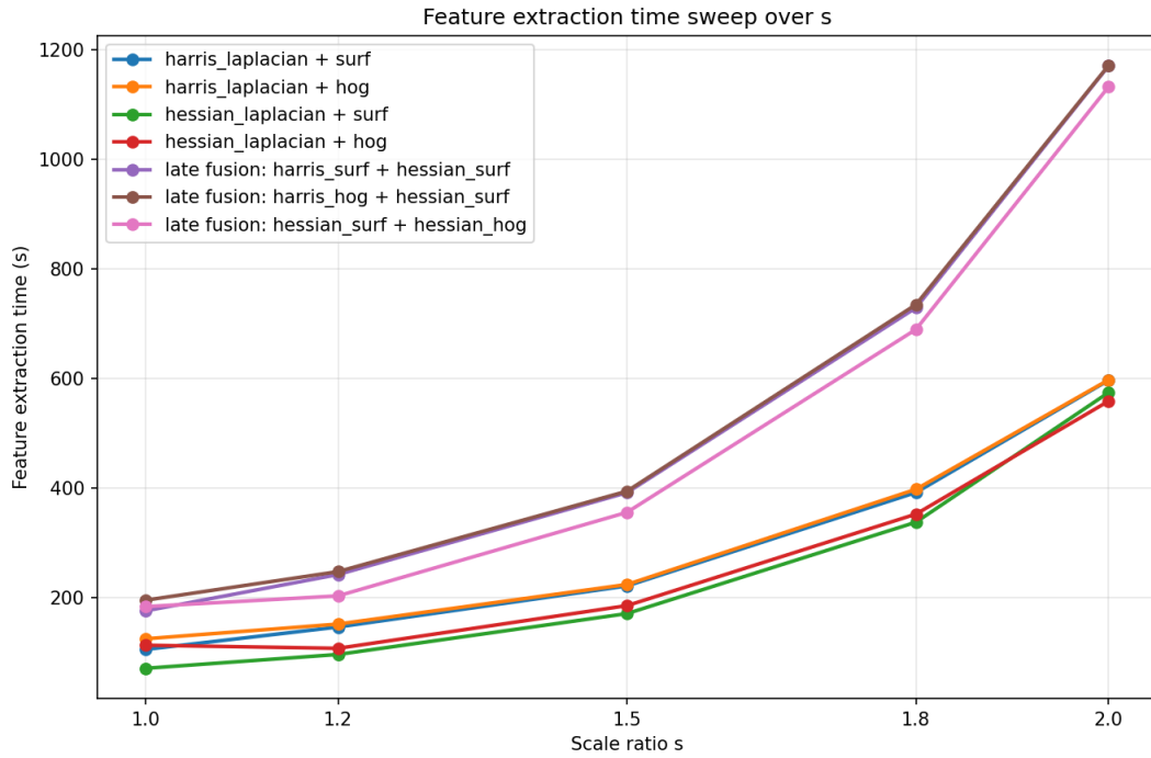
Σχήμα 46. Χρόνος εξαγωγής χαρακτηριστικών ως προς το s για όλους τους συνδυασμούς του Μέρους 3.1.
