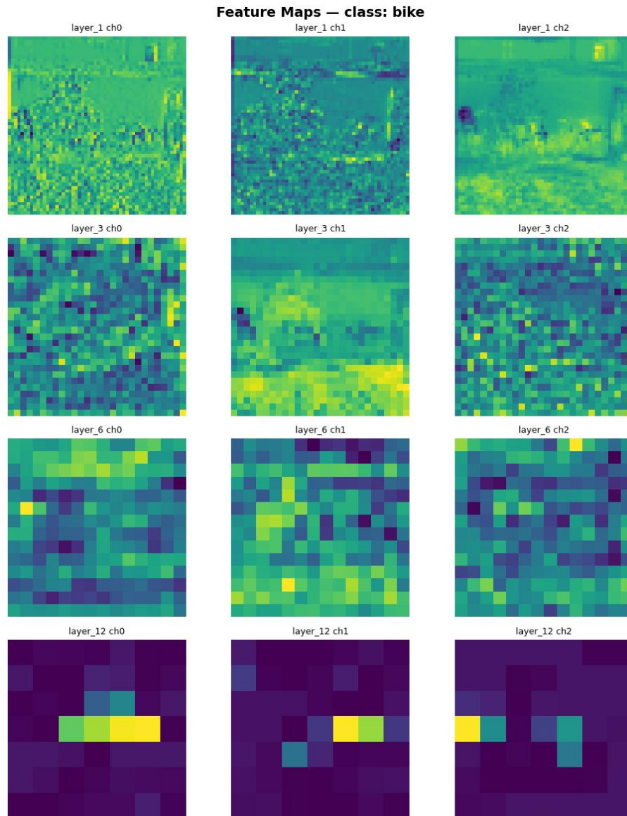
Σχήμα 52. Χάρτες ενεργοποίησης (3 κανάλια) για τα επίπεδα layer_1, layer_3, layer_6, layer_12 για τη κλάση: bike.
