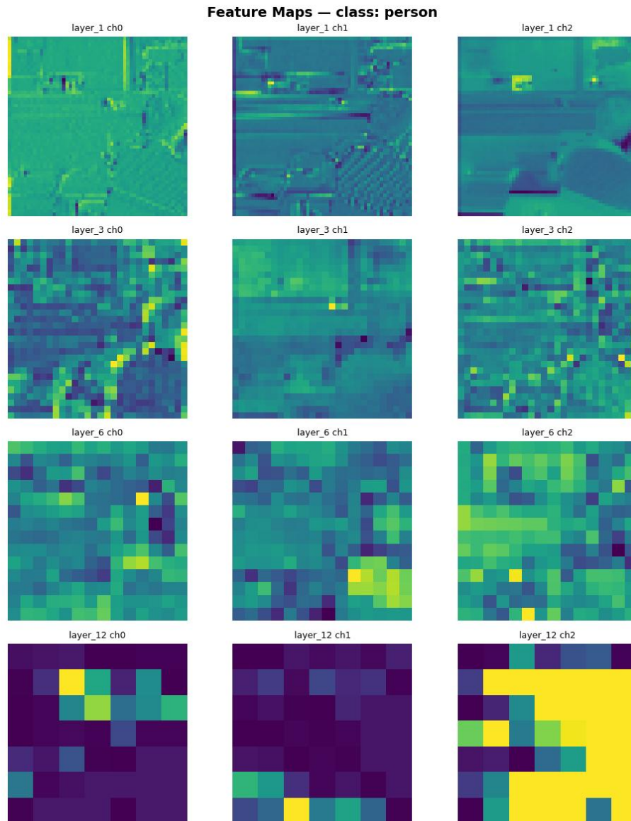
Σχήμα 51. Χάρτες ενεργοποίησης (3 κανάλια) για τα επίπεδα layer_1, layer_3, layer_6, layer_12 για τη κλάση: person.
