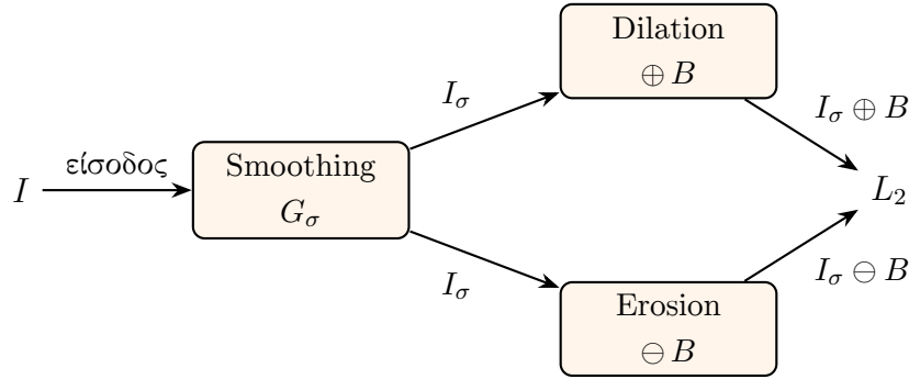
Σχήμα 5. Ροή υπολογισμού της μη-γραμμικής Laplacian L_2 : η εξομαλυσμένη εικόνα I_\sigma τροφοδοτεί παράλληλα τη dilation και την erosion, των οποίων τα αποτελέσματα συνδυάζονται ως (\oplus) + (\ominus) - 2I_\sigma .
