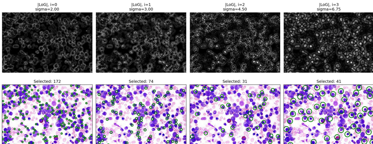
Σχήμα 32. Αντίστοιχη πολυκλιμακωτή οπτικοποίηση Harris-Laplacian για την blood_cells.jpg.
