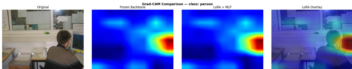
Σχήμα 55. Grad-CAM για κλάση person .
