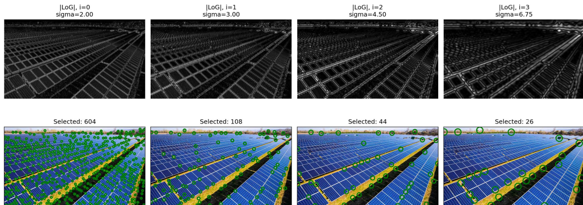
Σχήμα 40. Hessien-Laplace ανά κλίμακα για την solar.jpg. Η πρώτη γραμμή δείχνει την κανονικοποιημένη LoG, ενώ η δεύτερη τα blobs που παραμένουν μετά την επιλογή χαρακτηριστικής κλίμακας.
