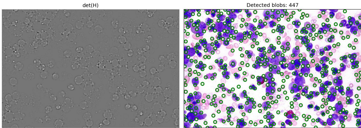
Σχήμα 37. Αποτελέσματα της ενότητας 2.3 για την εικόνα blood_cells.jpg. Ο ανιχνευτής Hessian ανταποκρίνεται έντονα στις σχεδόν κυκλικές δομές των κυττάρων, όπως αναμένεται από έναν blob detector.
