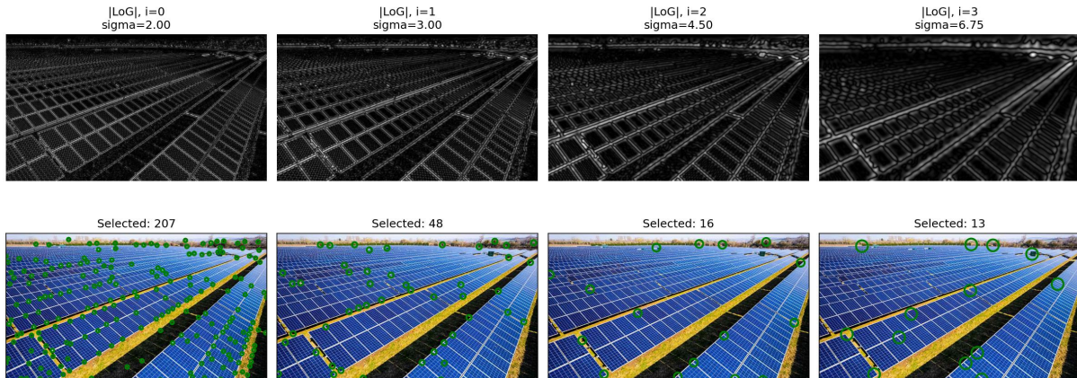
Σχήμα 31. Αναπαράσταση Harris-Laplacian ανά κλίμακα για τη solar.jpg. Η πρώτη γραμμή δείχνει την κανονικοποιημένη απόκριση LoG και η δεύτερη τα σημεία που διατηρούνται μετά τον έλεγχο μεγίστου ως προς την κλίμακα.
