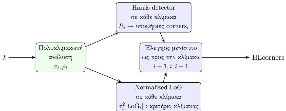
Σχήμα 35. Pipeline του αλγορίθμου Harris-Laplacian. Αρχικά εφαρμόζεται ο ανιχνευτής Harris σε πολλαπλές κλίμακες για την εύρεση υποψήφιων γωνιών και παράλληλα υπολογίζεται η κανονικοποιημένη LoG απόκριση. Τελικά διατηρούνται μόνο τα σημεία των οποίων η LoG απόκριση μεγιστοποιείται ως προς τις γειτονικές κλίμακες.
