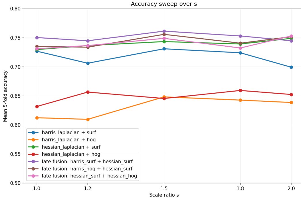
Σχήμα 45. Accuracy ως προς τον λόγο κλιμάκων s για όλους τους συνδυασμούς που υλοποιεί το part3_1.py.
