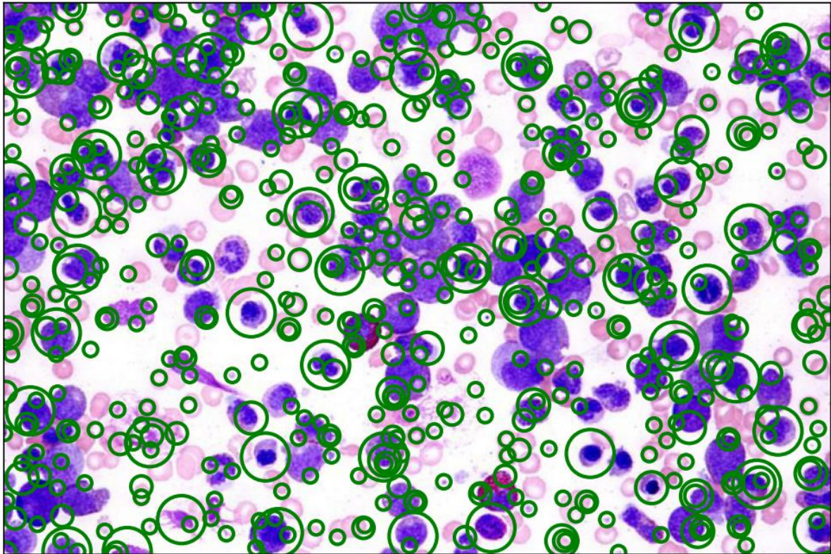
Σχήμα 43. Τελικά blobs Hessian-Laplace για την εικόνα blood_cells.jpg.
