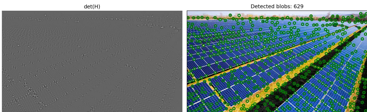
Σχήμα 36. Αποτελέσματα της ενότητας 2.3 για την εικόνα solar.jpg . Αριστερά φαίνεται η απόκριση \det(H) και δεξιά τα blobs που εντοπίστηκαν σε μία μόνο κλίμακα.
