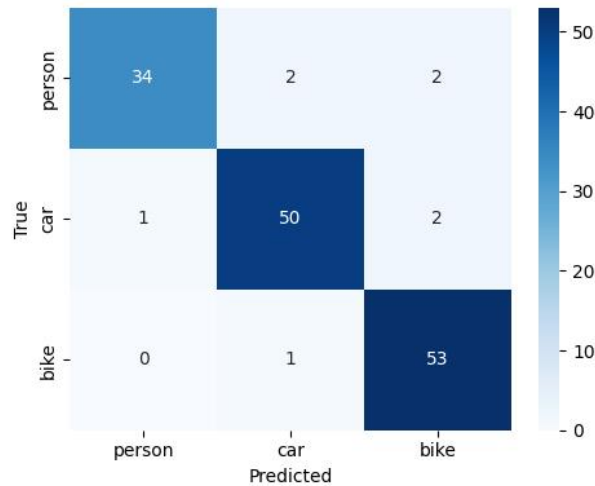
Σχήμα 49. Confusion Matrix του MobileNetV3-Small + SVM στο test set. Κάθε γραμμή αντιστοιχεί στην αληθινή κλάση και κάθε στήλη στην προβλεπόμενη.
