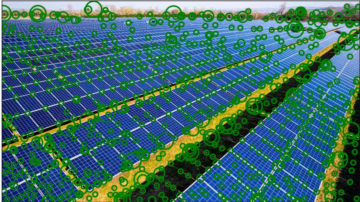
Σχήμα 42. Τελικά blobs Hessian-Laplace για την εικόνα solar.jpg.
