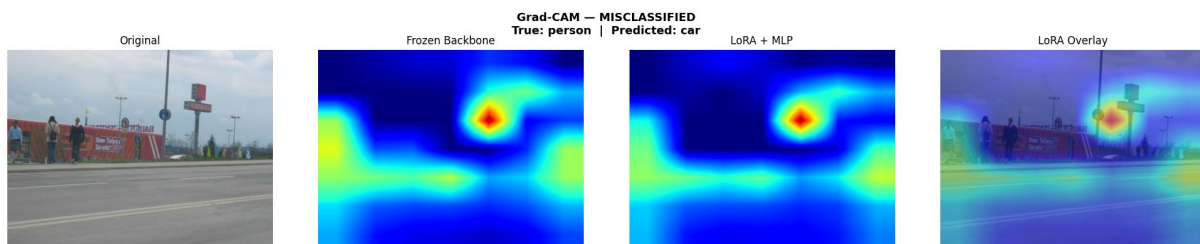
Σχήμα 58. Grad-CAM για λανθασμένα ταξινομημένο δείγμα: αληθινή κλάση person , προβλεπόμενη car . Ο χάρτης CAM εστιάζει στον δρόμο και τη σήμανση αντί στον άνθρωπο.
