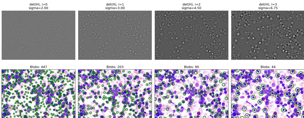
Σχήμα 39. Πολυκλιμακωτή απόκριση \det(H) και τα αντίστοιχα blobs για την blood_cells.jpg πριν από την επιλογή της τελικής χαρακτηριστικής κλίμακας.
