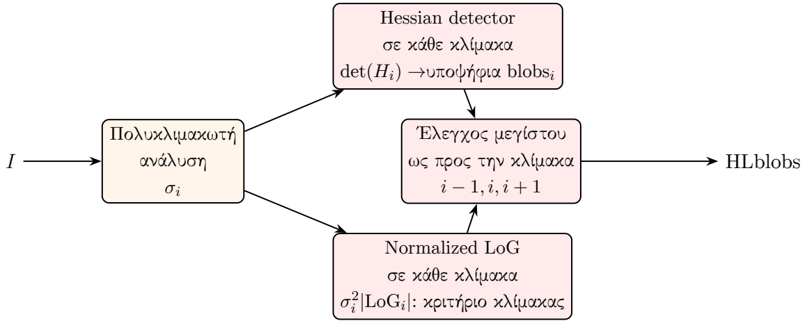
Σχήμα 44. Pipeline του αλγορίθμου Hessian-Laplace. Αρχικά εφαρμόζεται ο ανιχνευτής Hessian σε πολλαπλές κλίμακες για την εύρεση υποψήφιων blobs και παράλληλα υπολογίζεται η κανονικοποιημένη LoG απόκριση. Τελικά διατηρούνται μόνο τα σημεία των οποίων η LoG απόκριση μεγιστοποιείται ως προς τις γειτονικές κλίμακες.
