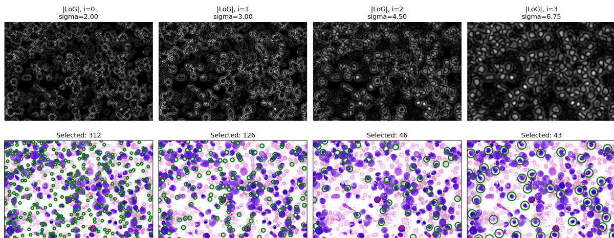
Σχήμα 41. Αντίστοιχη διαδικασία για την blood_cells.jpg. Ο ανιχνευτής Hessien-Laplace επιλέγει κυρίως τις σχεδόν κυκλικές δομές των κυττάρων στις κλίμακες όπου εμφανίζονται πιο σταθερές.
