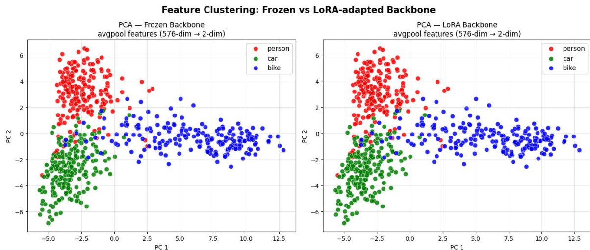
Σχήμα 54. PCA (με 2 διαστάσεις) των avgpool χαρακτηριστικών 576-dim για τον frozen backbone (αριστερά) και τον LoRA-aligned (δεξιά).
