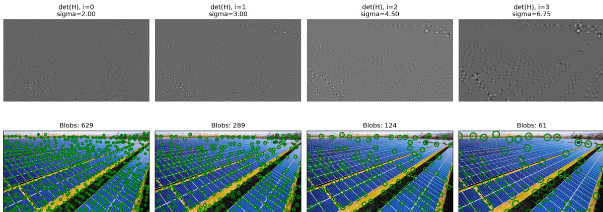
Σχήμα 38. Πολυκλιμακωτή απόκριση \det(H) και τα αντίστοιχα blobs για την solar.jpg πριν από το στάδιο επιλογής χαρακτηριστικής κλίμακας.
