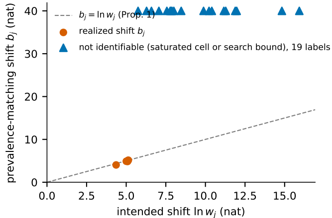
A. Realized vs. intended shift per label
