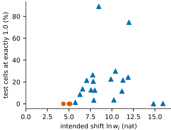
B. Saturation per label
