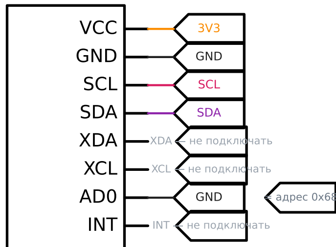
IMU MPU6050 (GY-521, без магнит.)
