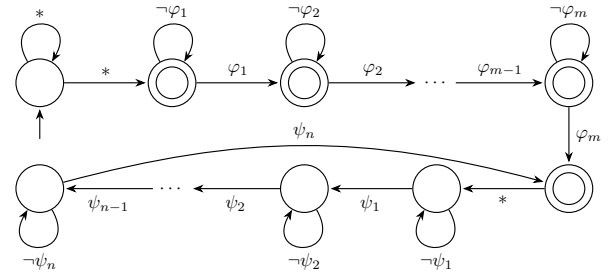
Fig. 7: GR(1) automaton.
