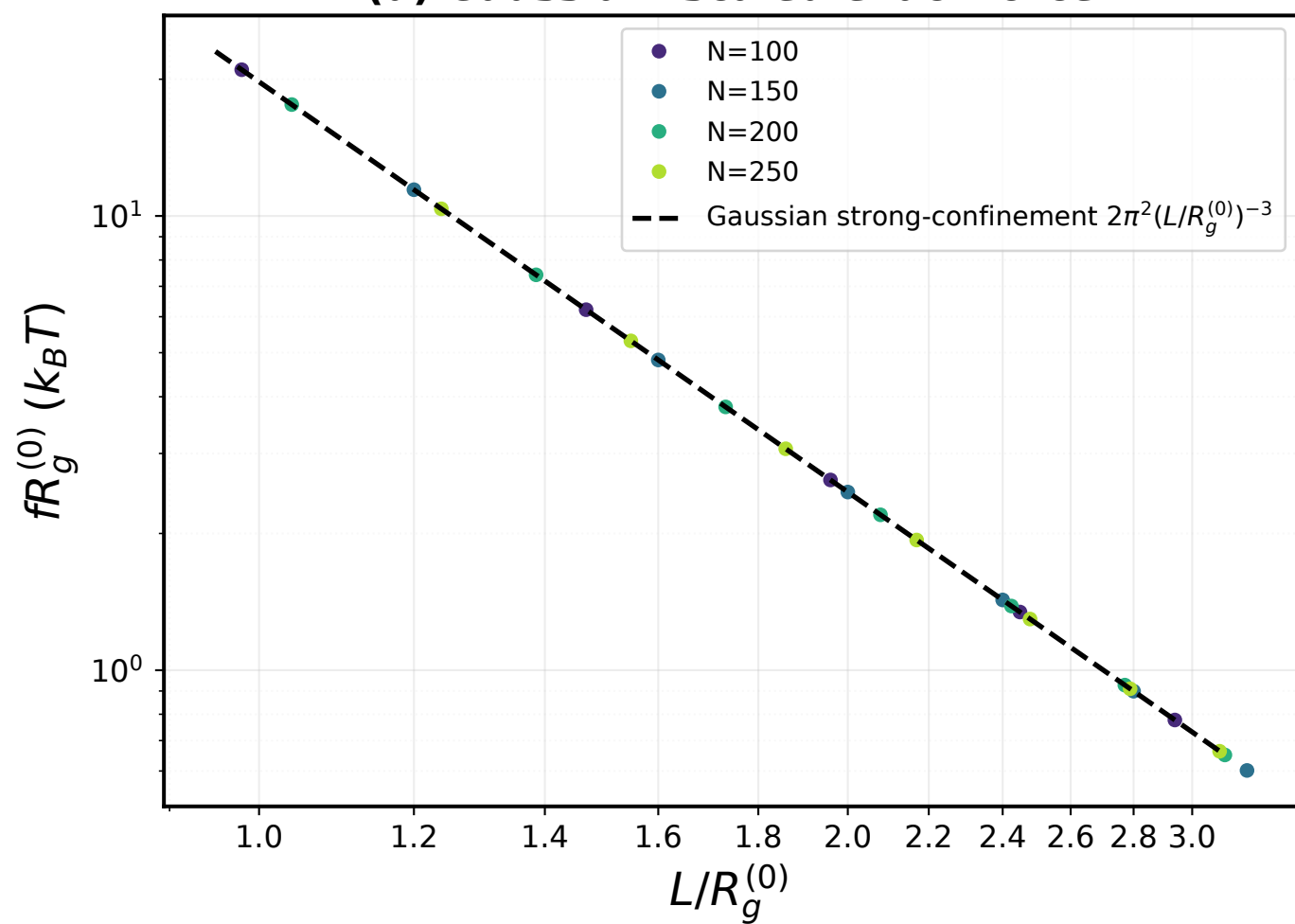
(d) Gaussian: scaled exact force
