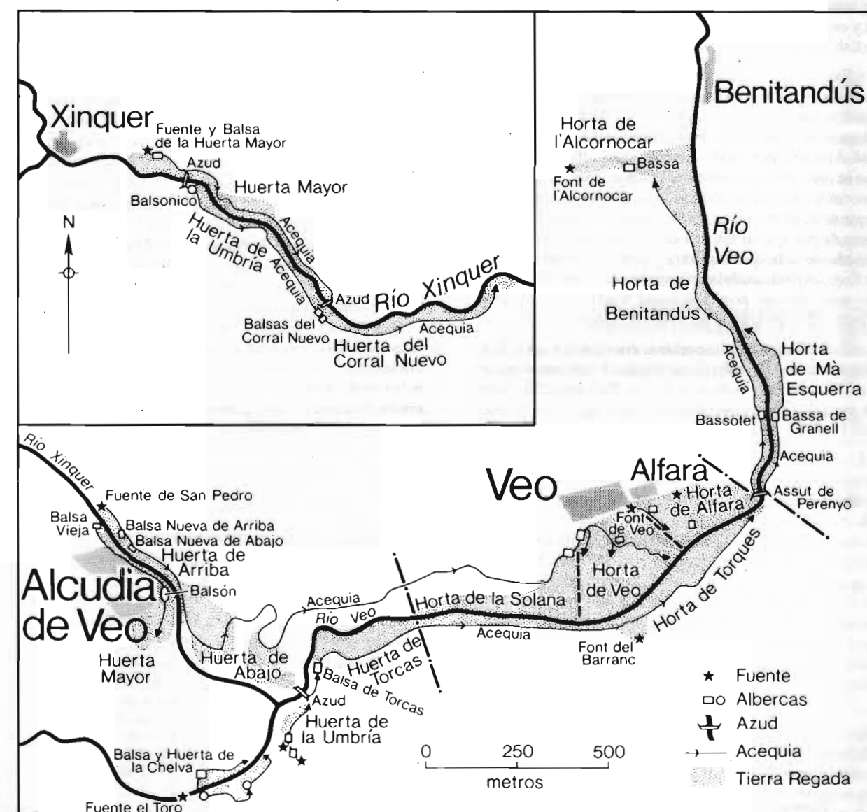
Fig. 2. Sistemas de regadío de la Vall de Veo
