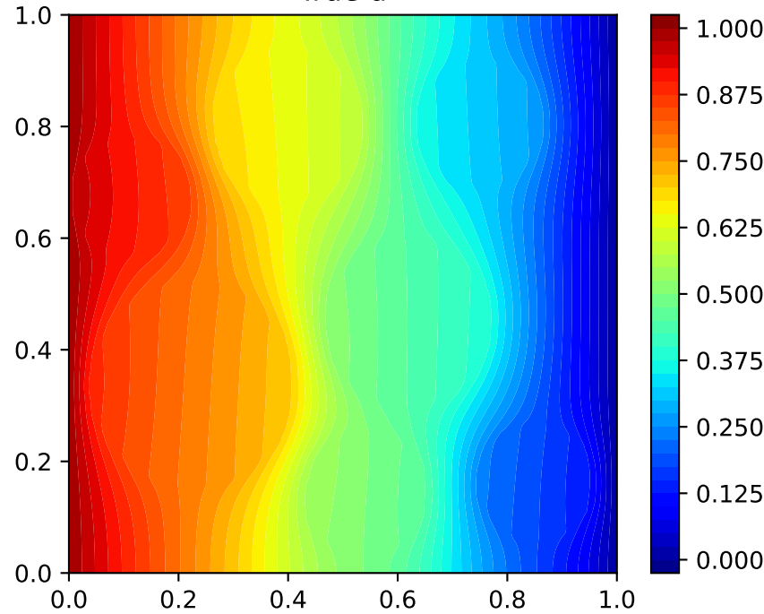
True u
