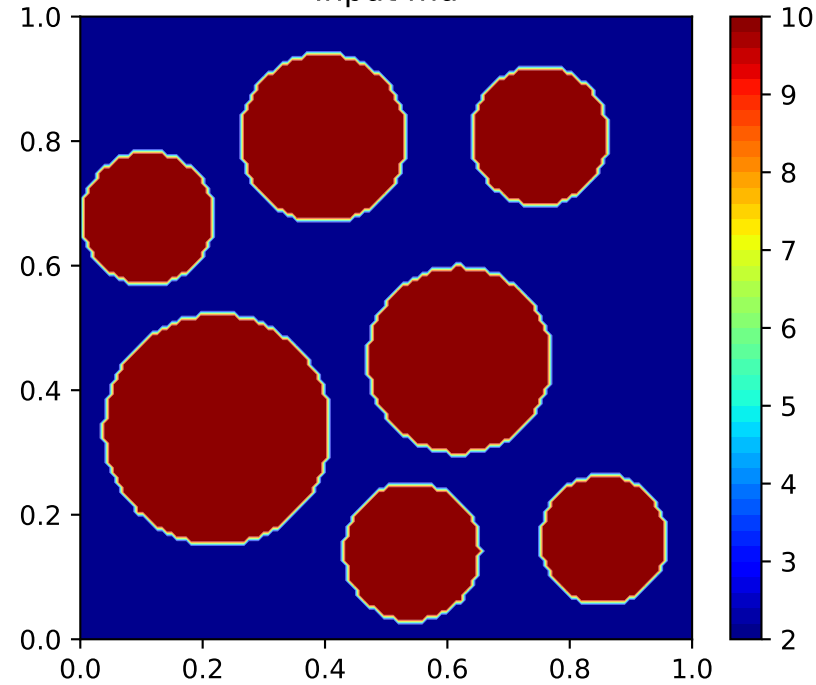
Input \mu
