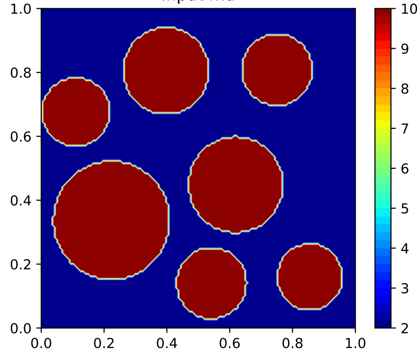
Input \mu
