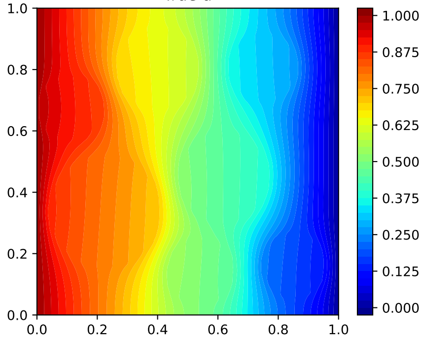
True u
