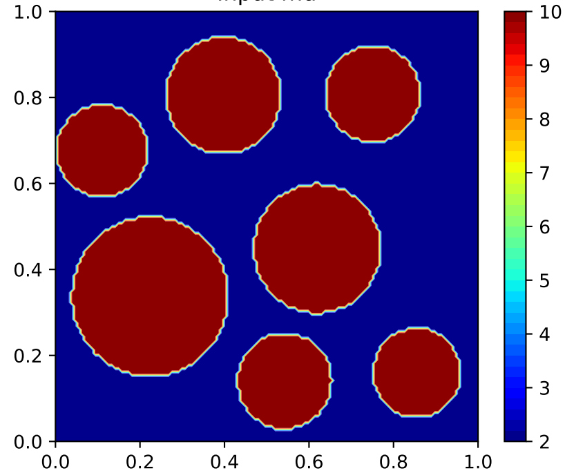
Input \mu
