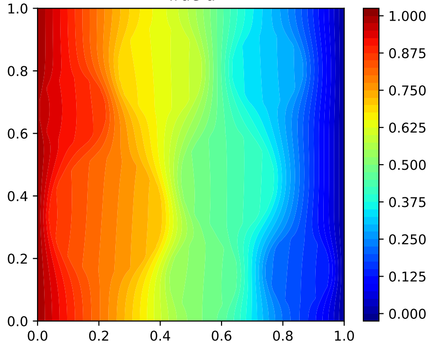
True u
