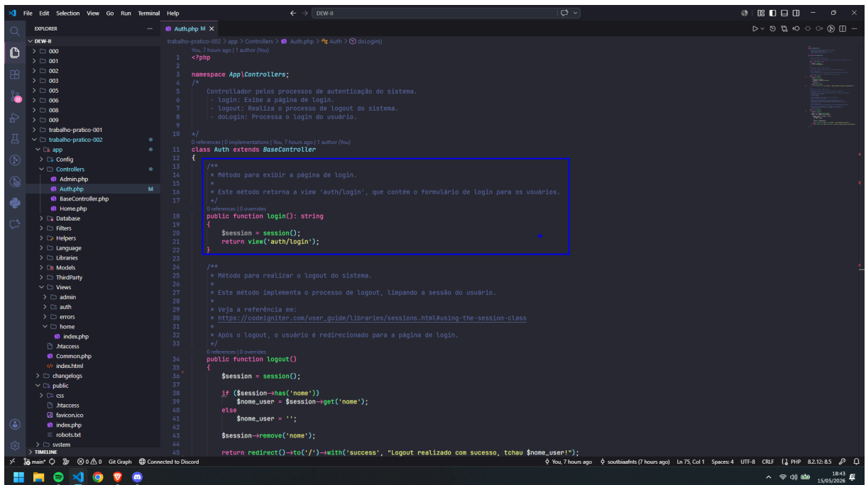
Figura 2 - Auth::login
