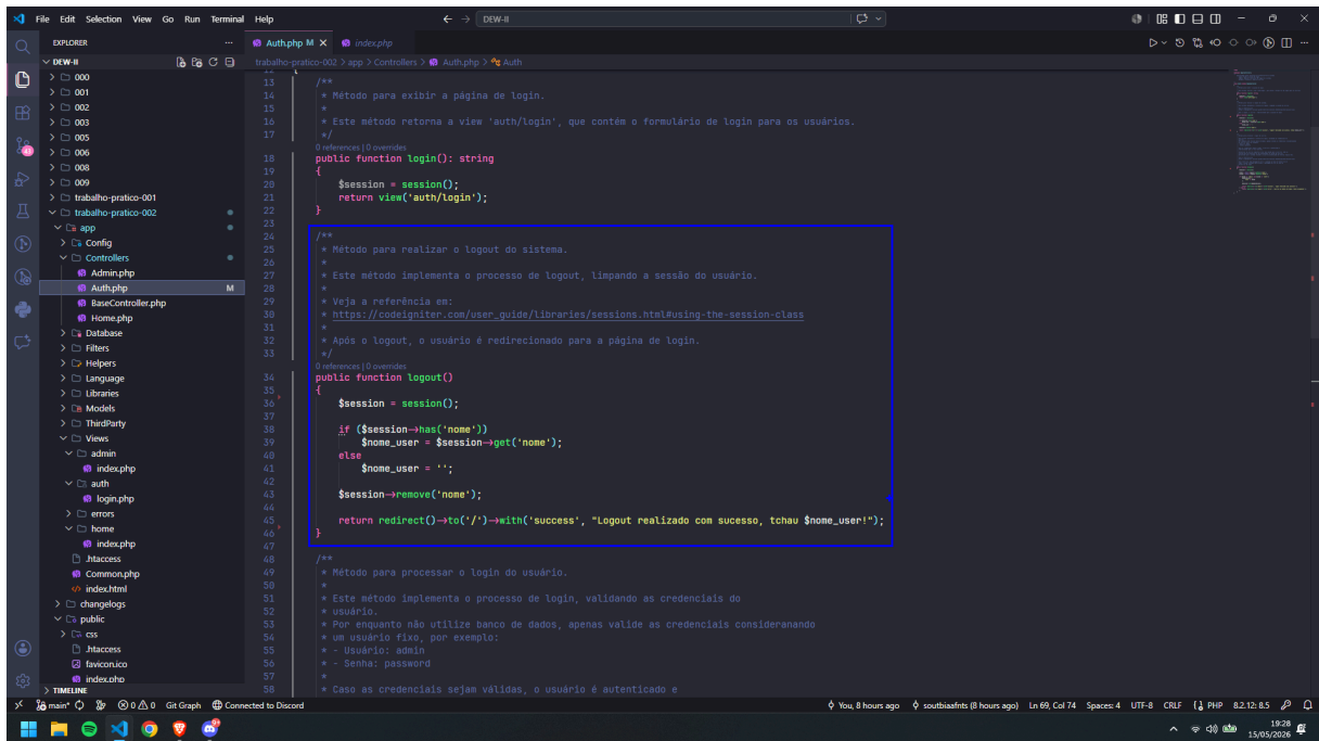
Figura 4 - Auth::logout
