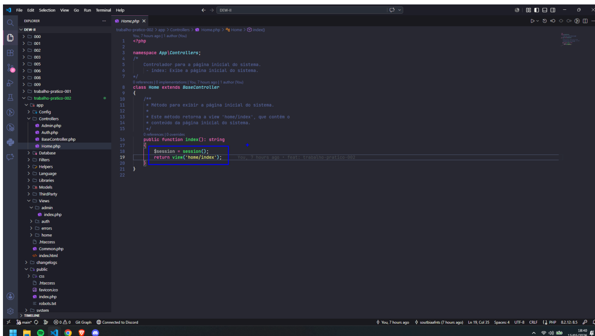
Figura 1 - Controlador Home
