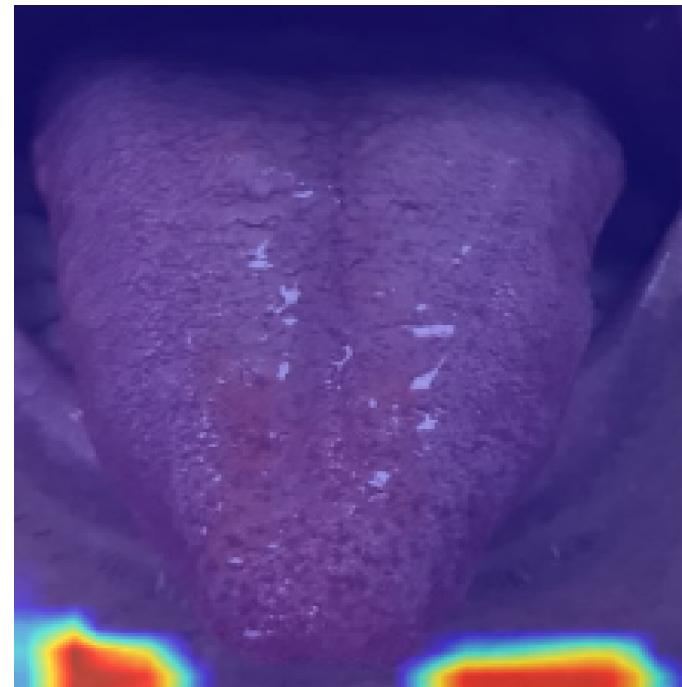
FFTran (SOTA)
