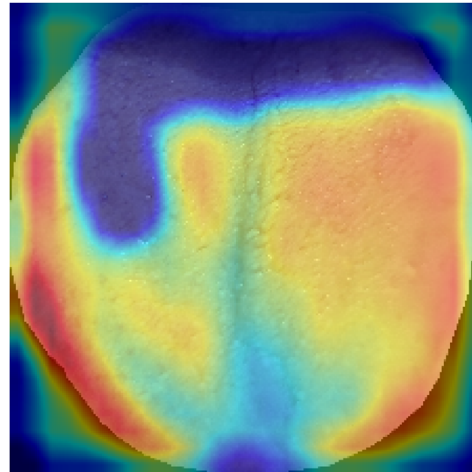
FFTran (SOTA)
