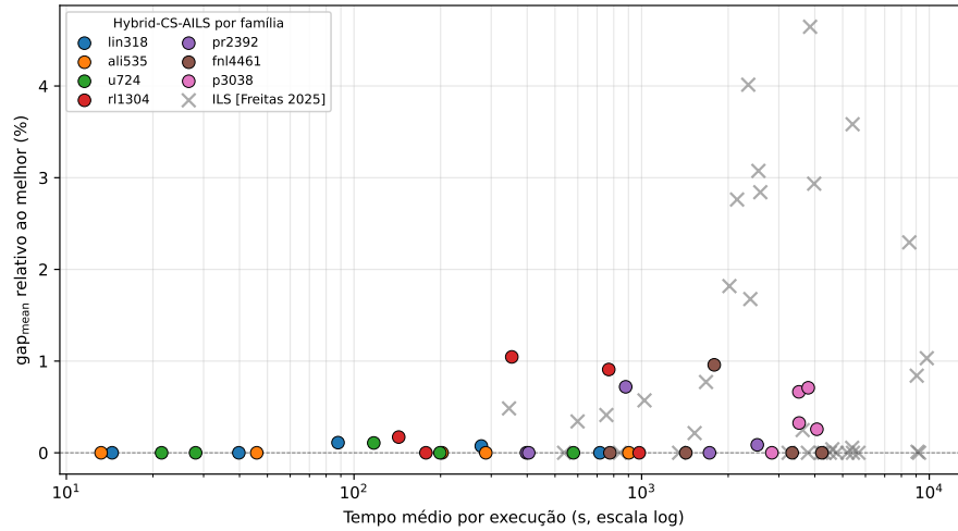
Figura 2: Fronteira tempo \times qualidade entre Hybrid-CS-AILS e ILS Freitas et al. [2025] sobre as 35 instâncias. Cada ponto representa o tempo médio por execução de uma instância; para o ILS, os valores são os reportados na publicação original. O eixo y é o gap percentual do custo médio em relação ao melhor entre os dois métodos em cada instância.
