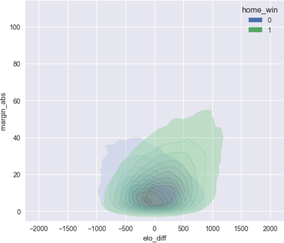
Density: elo_diff × margin_abs
