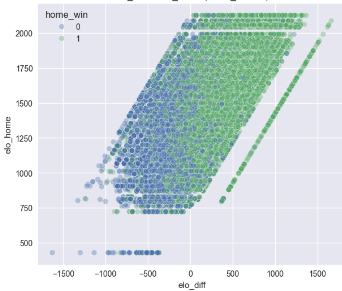
elo_diff vs elo_home (home_win 0/1)
