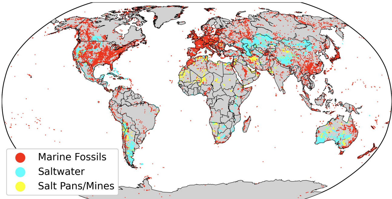
Figure 2. 전 세계의 해양(해양) 화석, 염수, 및 염전/염광의 분포 [34, 78, 67, 27].
