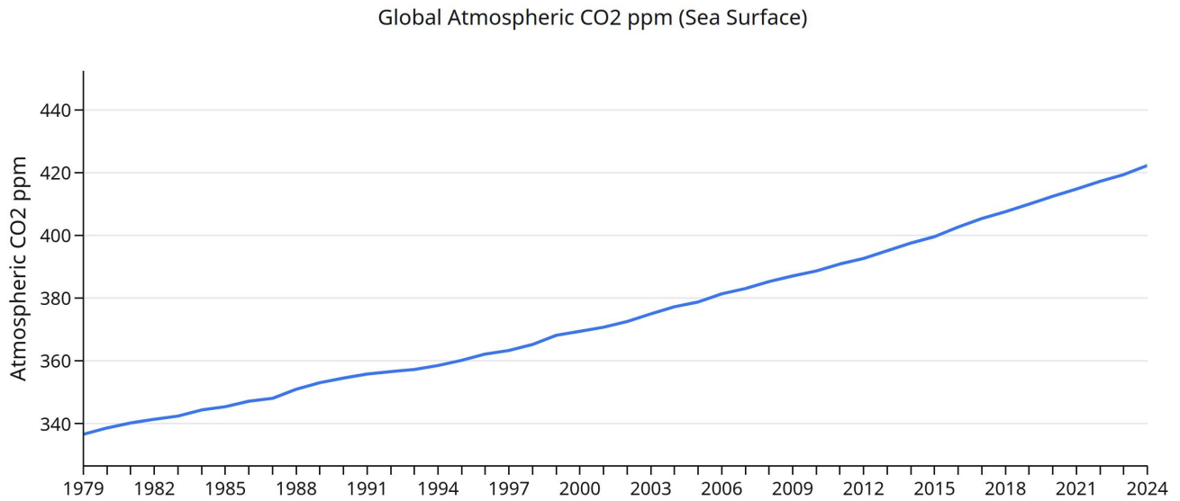
Figure 21. 지난 45년 동안 꾸준히 증가한 대기 중 CO2 농도. 이는 해양 온도의 상승으로 인해 발생했을 가능성이 높음. 출처: NOAA [33, 65].
