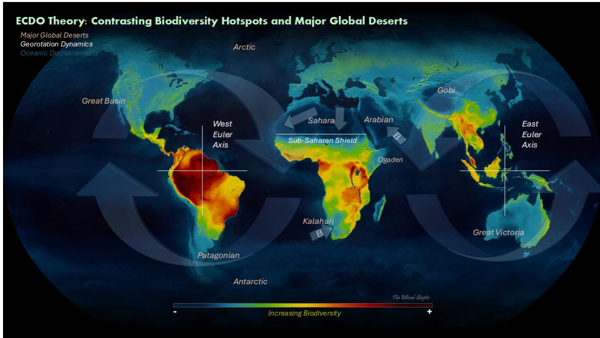
Figure 7. 세계 주요 사막과 교차하는 생물 다양성 핫스팟 [56]
