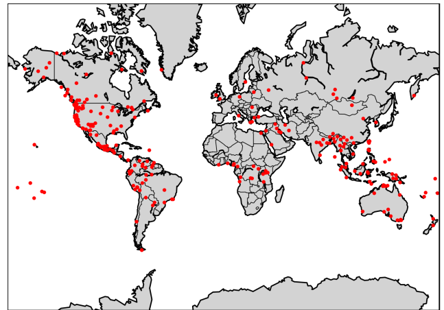
Figure 1. 전 세계의 홍수 이야기 위치 [64].
