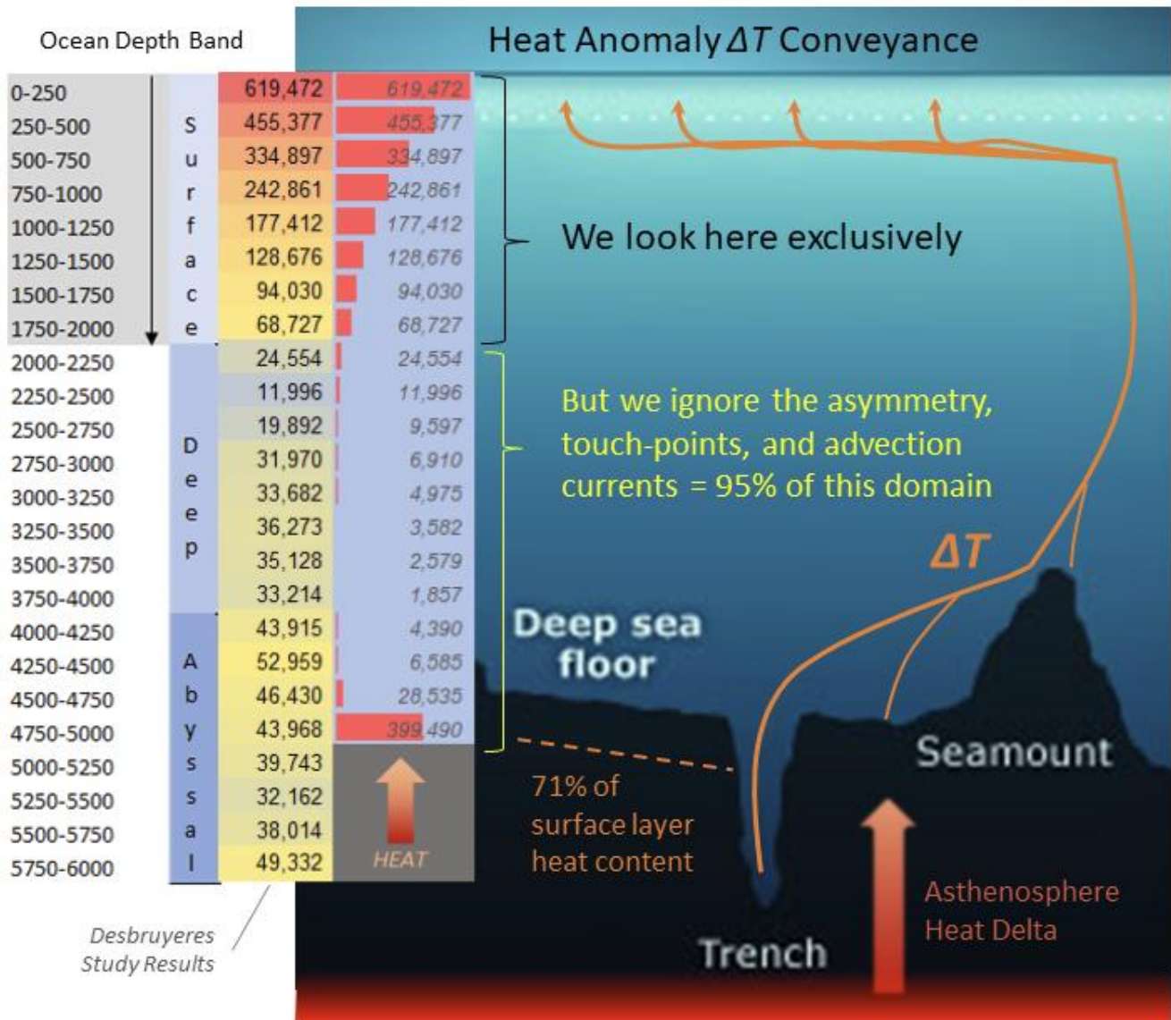
Figure 19. 대기의 작용에 의한 정상적인 해양 가열 곡선과 비교한 심해층 및 심해대의 해양 이상 가열 현상의 시각화. NOAA의 전체 이상 가열 현상 자료는, [36], Desbruyeres의 심해 및 심해 가열 분포 연구자료 및 [13], Ethical Skeptic의 데이터 처리 및 시각화 자료를 인용했다. [65].
