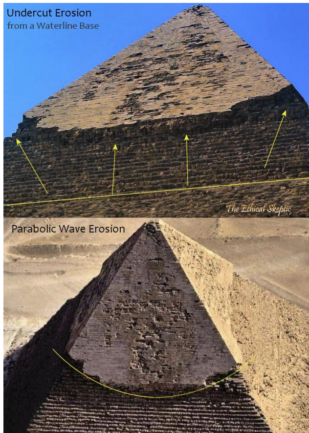
Figure 17. 카프레 피라미드에 있는 포물선형 하부 침식에 대한 자세한 관찰 [57].
