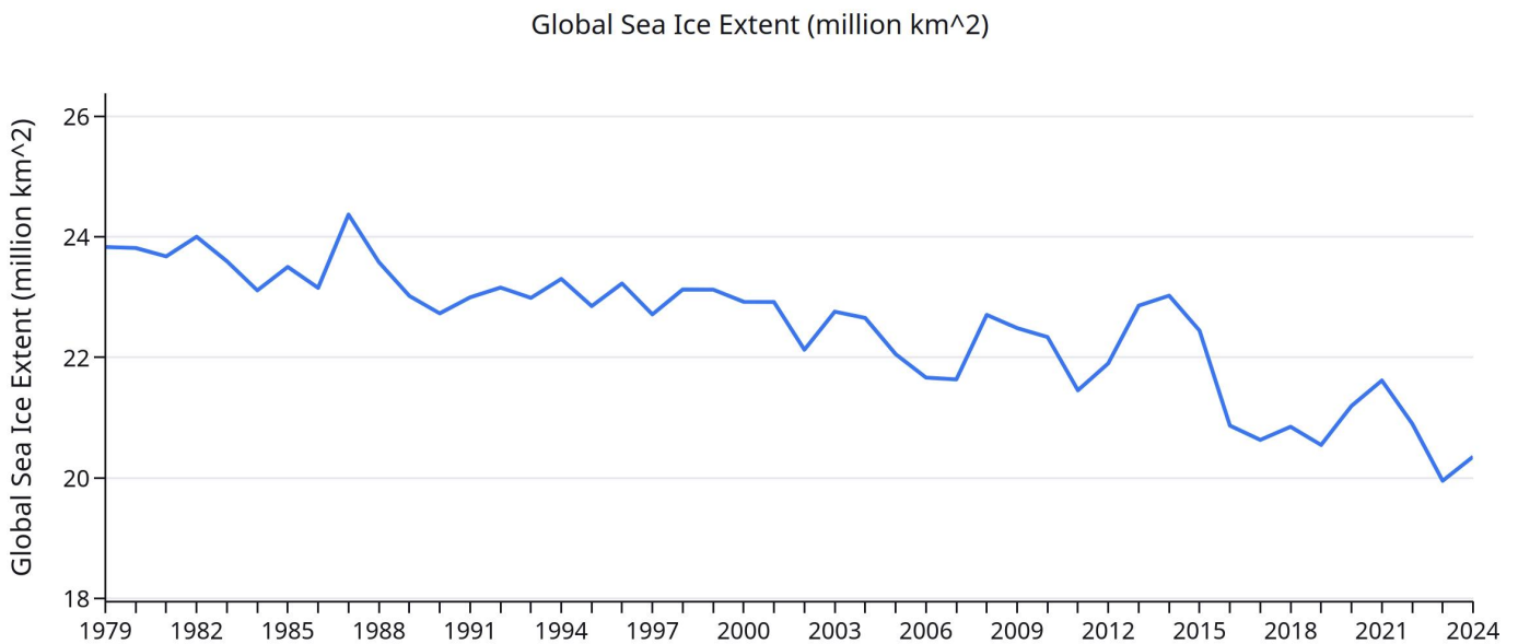
그림 22. 지난 45년 동안 지구의 온난화로 인해 줄어들고 있는 지구 해빙 면적. 출처: ADS [3].
