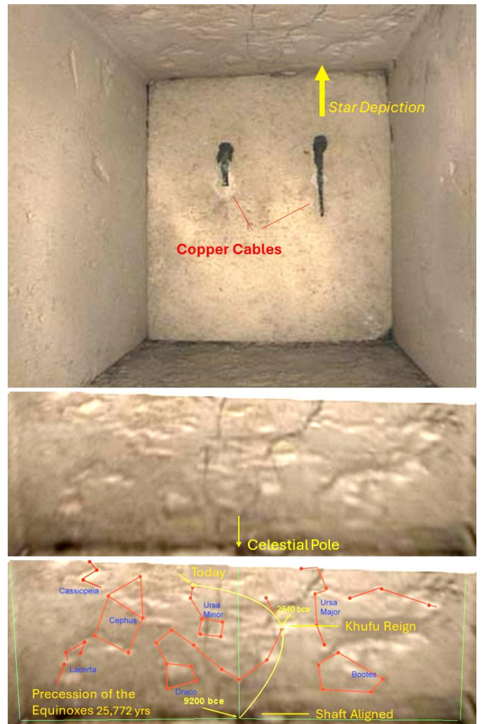
그림 18. 쿠푸 피라미드의 한 통로에 새겨진 별 지도 [56].
