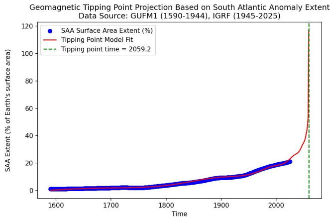
그림 16. 남대서양 이상 현상을 기반으로 계산된 특이한 결정적 전환점, 2059년 3월 13일 [24, 48].
