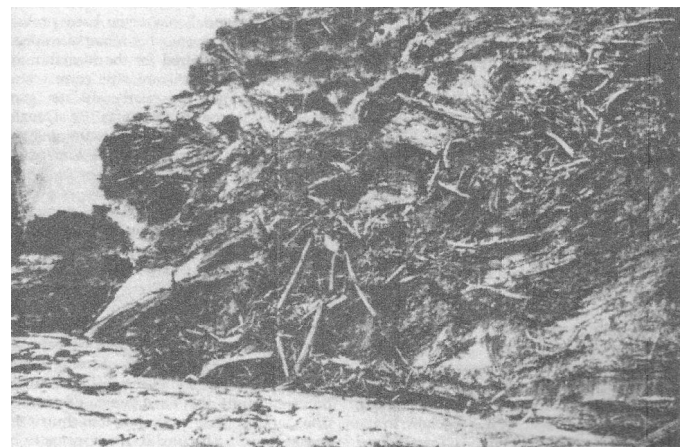
그림 7. 냉동 실트와 얼음 속에 나무, 식물 및 동물 조각이 어지럽게 흩어져 있는 알래스카의 '머크' [57].
