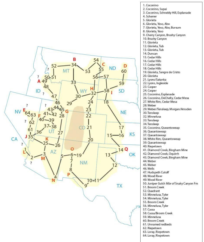
그림 3. 미국 서부에 있는 코코니노 사암 층의 크기 [62].
