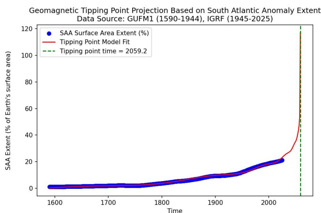
图 16. 基于南大西洋异常的一个临界点计算得出日期为 2059 年 3 月 13 日 [25, 49]。
