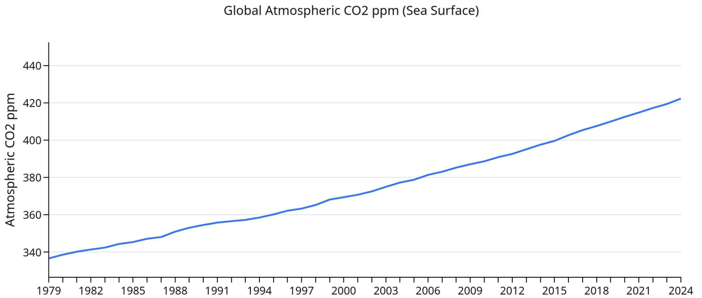
图 21. 大气中的二氧化碳浓度在过去的 45 年中持续上升，可能是由于海洋温度的升高引起的。来源：NOAA [34, 66]。
