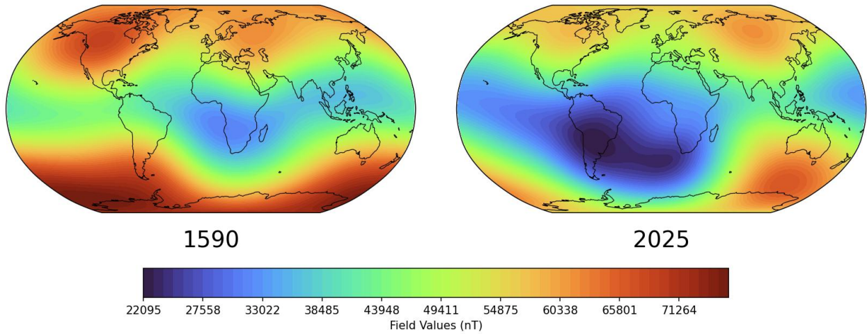
图 12. 从 1590 年到 2025 年的地磁场削弱的描述。使用 gufm1 和 IGRF-14 模型计算 [25, 49]。
