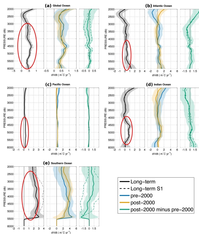
图 15. 1991 年到 2010 年深 (>2000 米深度) 海洋变暖率, 红色圆圈标出 [14]。
