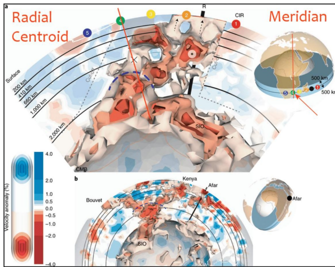
图 13. 南非下方 LLVP 的详细视觉 [57]。
