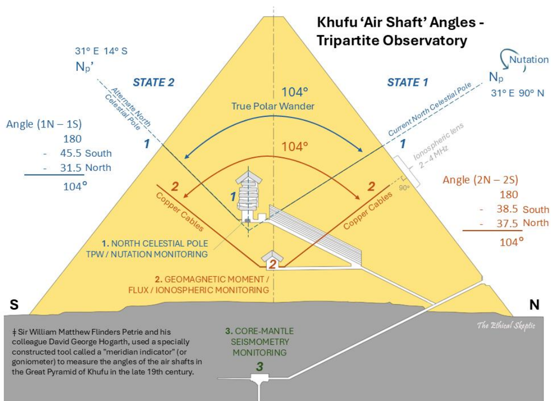
图 5. 胡夫金字塔的内部通道和房间，Ethical Skeptic 提议这是一个用于 ECDO 事件的三部分地球物理监测天文台 [57]。
