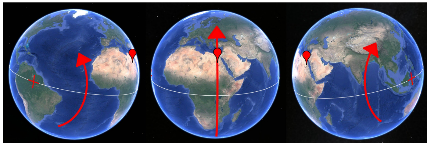
图 6. 提议的 ECDO 旋转示意图，沿 31 度东经以北 104 度旋转，十字标记显示东西支点，红色标记显示胡夫金字塔。
