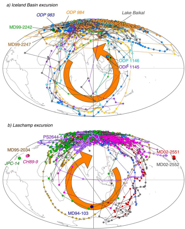
图 8. (a) 冰岛盆地偏移和 (b) 拉尚普偏移的虚拟地磁极轨道 [33]
