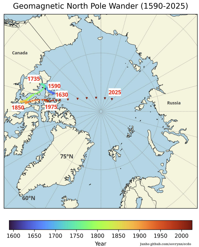
图 14. 1590 年至 2025 年地磁北极位置，每 5 年增量描述 [48]。
