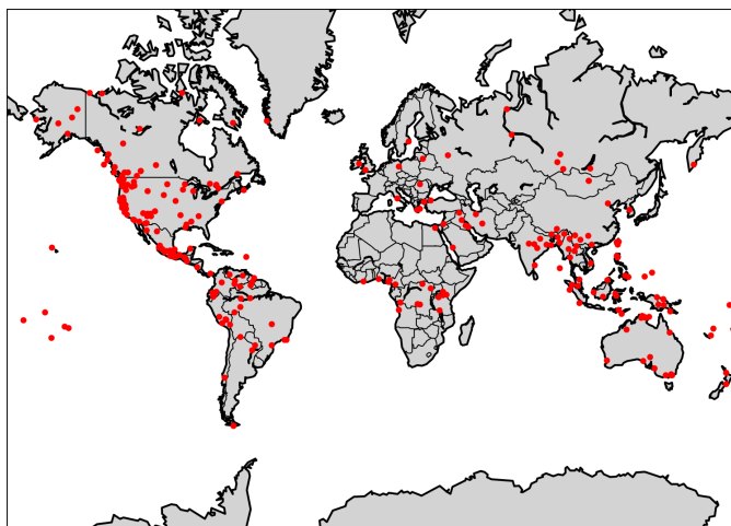
图 1. 世界各地洪水传说的起源地 [65]
