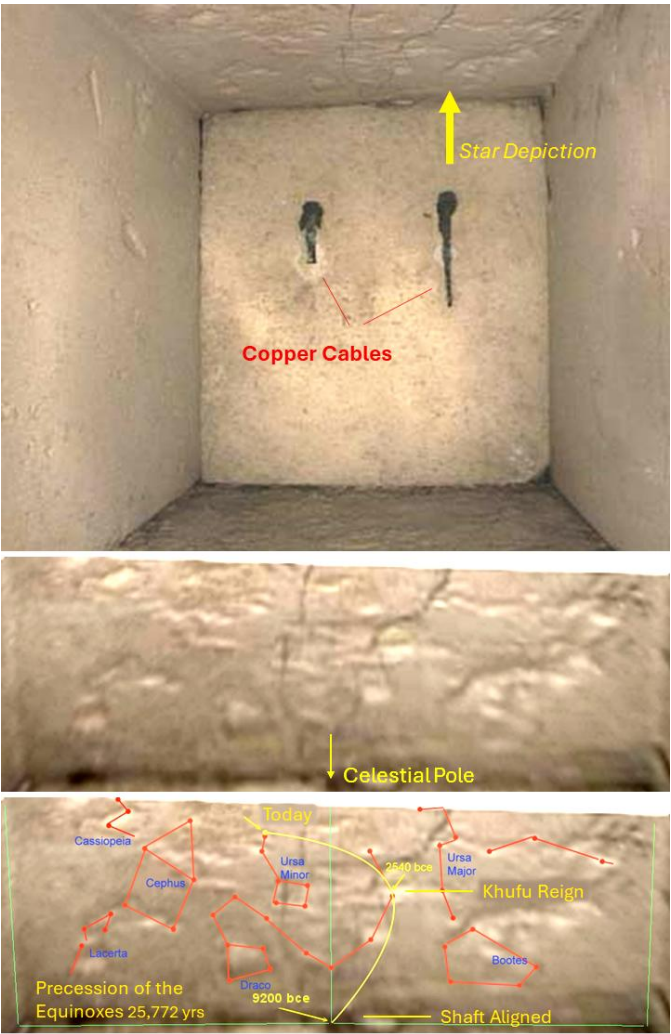
图 18. 在胡夫金字塔的一个通道中刻在石头上的星图 [57]。
