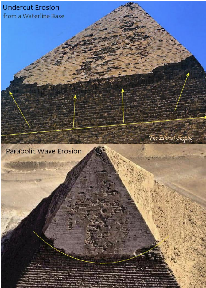
图 17. 近距离观察哈夫拉金字塔上的底切抛物线波侵蚀 [58]。
