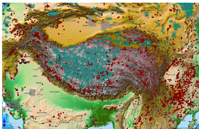
图 3. 显示盐水 (青)、干盐 (白) 和海洋化石 (红色) 的喜马拉雅地形图 [35, 79, 68, 28]。
