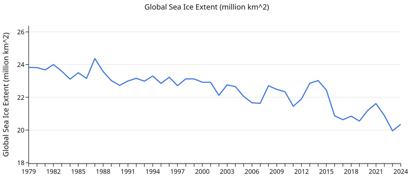
图 22. 全球海冰范围在过去的 45 年中一直在缩小，这归因于地球变暖。来源：ADS [3]。
