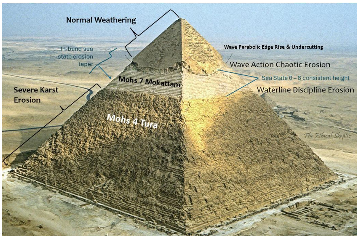
图 4. 显示由持续的暂时海平面上升造成的差异性、图案化喀斯特侵蚀的示意图 [58]。
