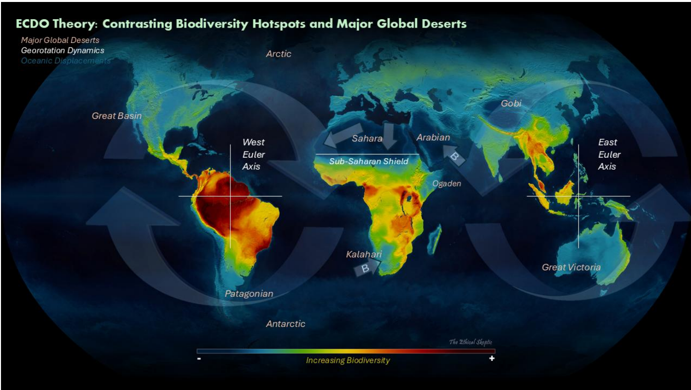
图 7. 世界主要沙漠和交替的生物多样性热点示意图 [57]。
