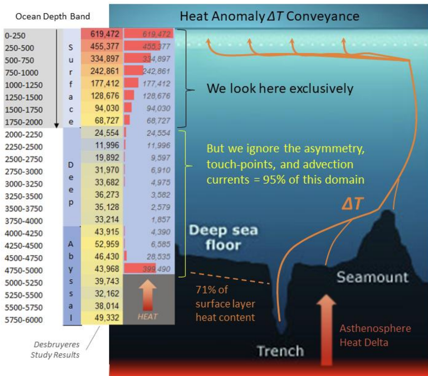
图 19. 深海和深海底加热异常与正常大气海洋加热曲线的对比视觉效果。整体加热异常来自 NOAA [37]，深海和深海底加热分布来自 Desbruyeres 研究 [14]，数据处理和可视化由 Ethical Skeptic 完成 [66]。
