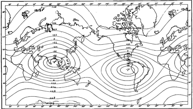
图 9. 地壳中的剪切模式示意图 [43]。
