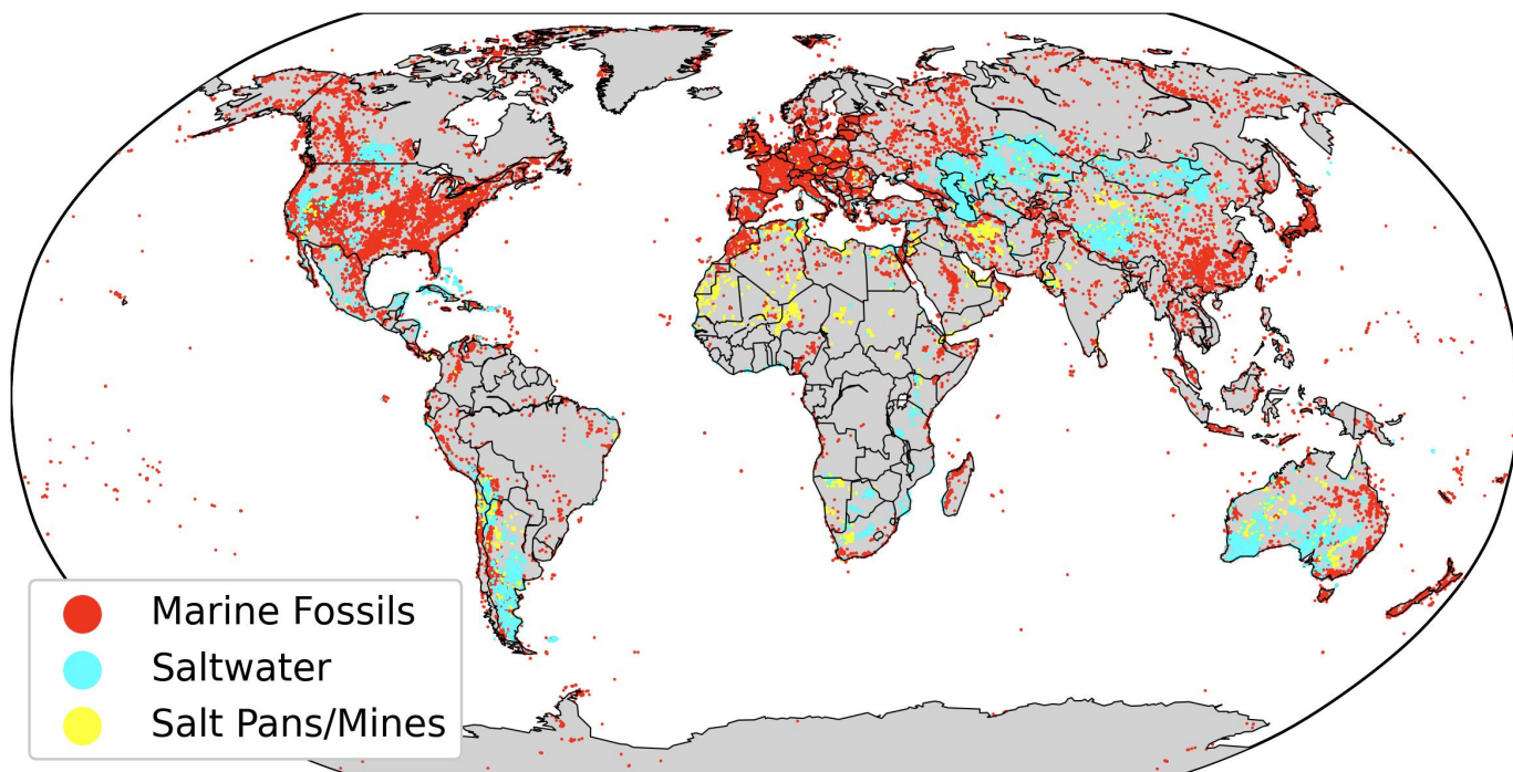
图 2. 全球海洋化石、咸水和盐滩/矿井分布图 [35, 79, 68, 28]。
