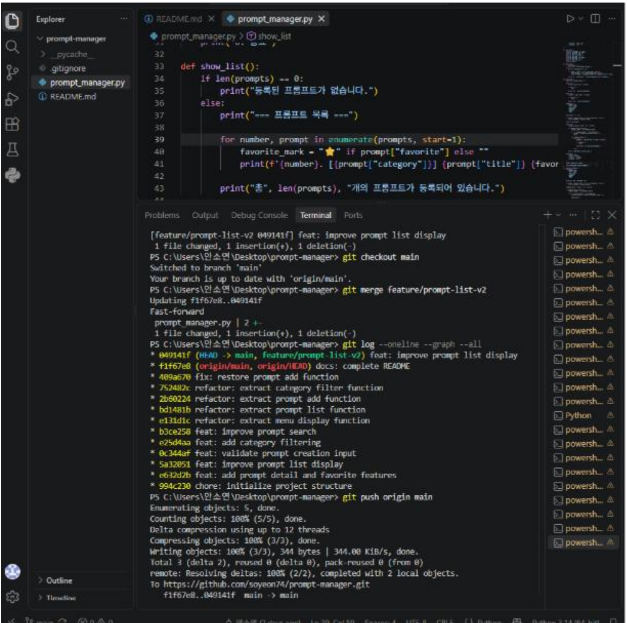
그림 7. 제출 중병 당시 기능 단위 커밋 13개 및 GitHub push 결과
