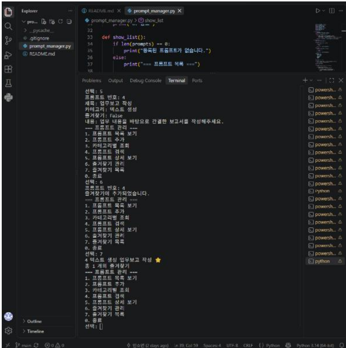
그림 6. 상세 보기, 즐겨찾기 상태 변경 및 즐겨찾기 목록 확인
