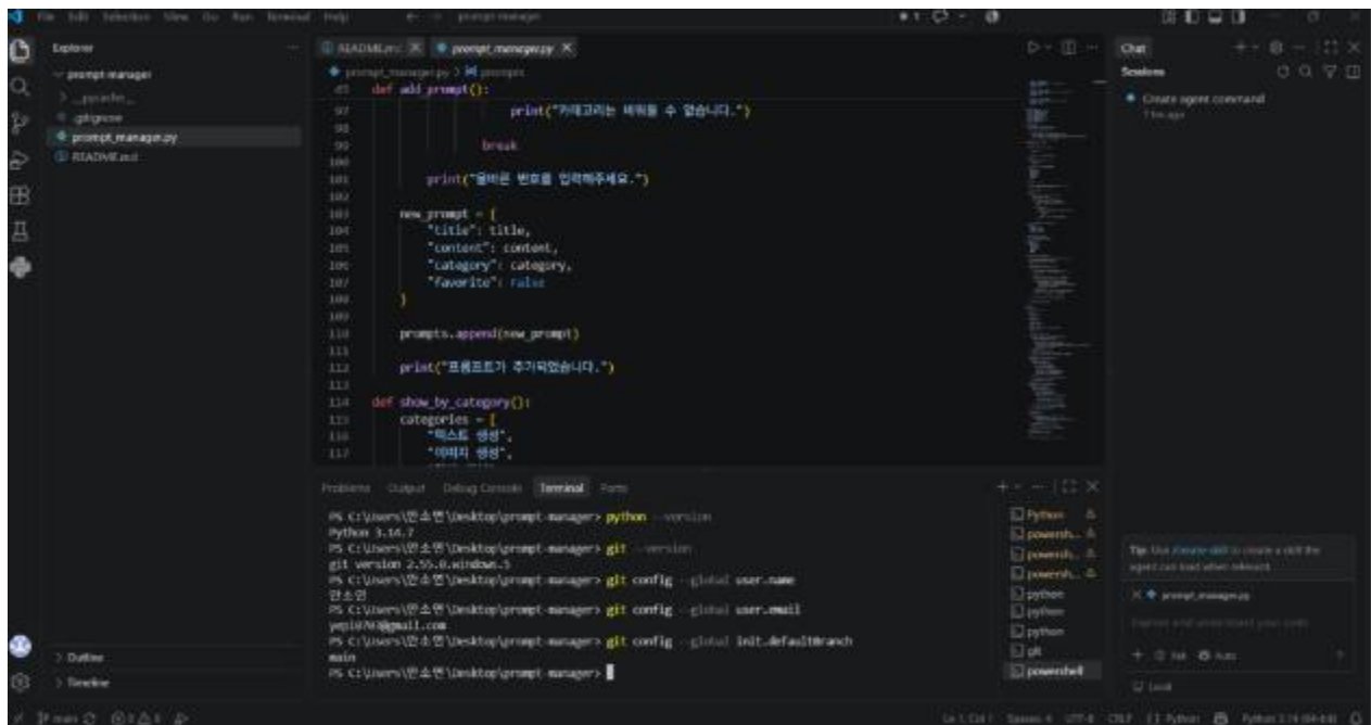
그림 1. Python-Git 버전 및 Git 사용자/기본 브랜치 설정 확인
