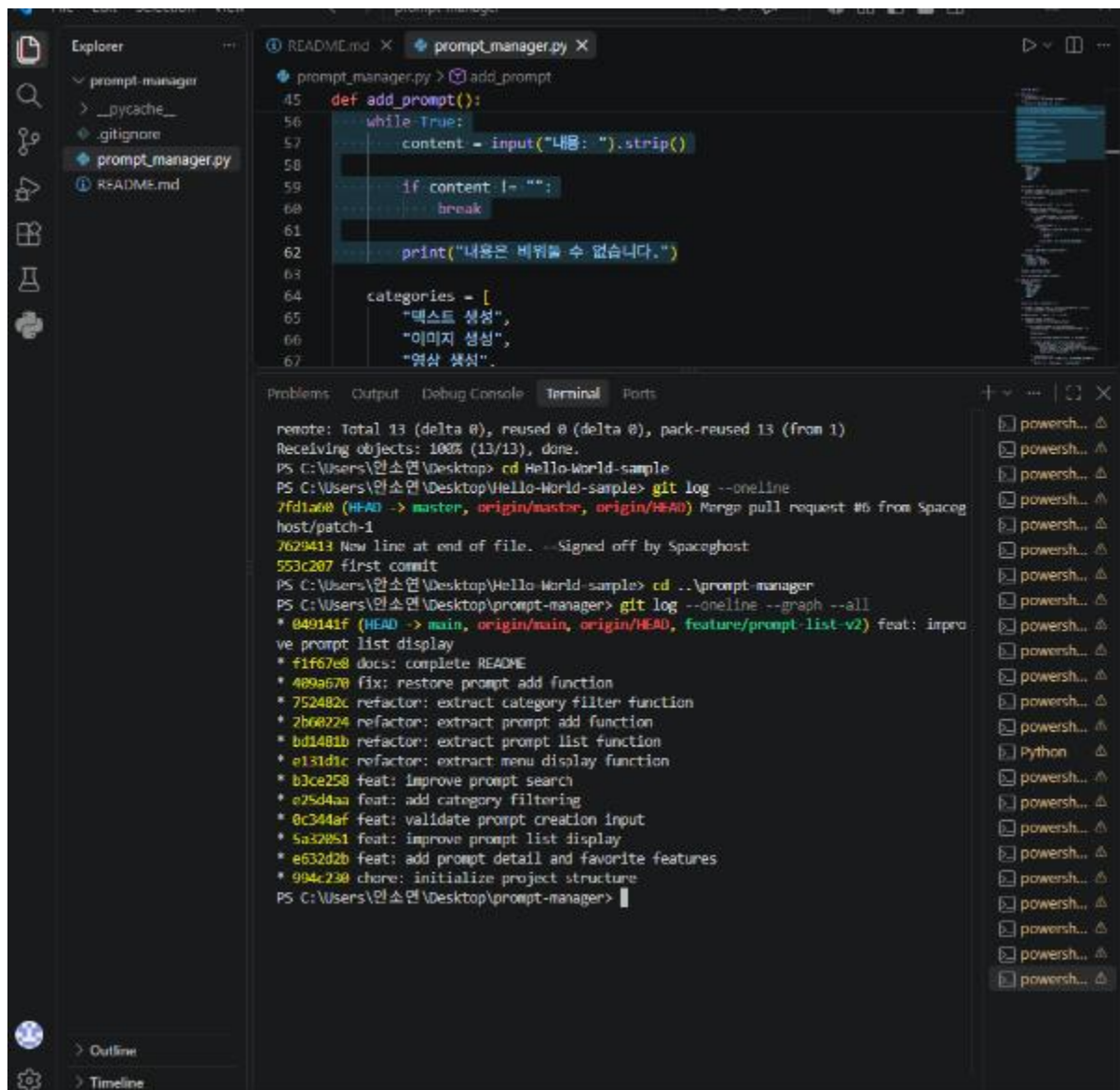
그림 8. git log --oneline --graph --all 최종 기록
