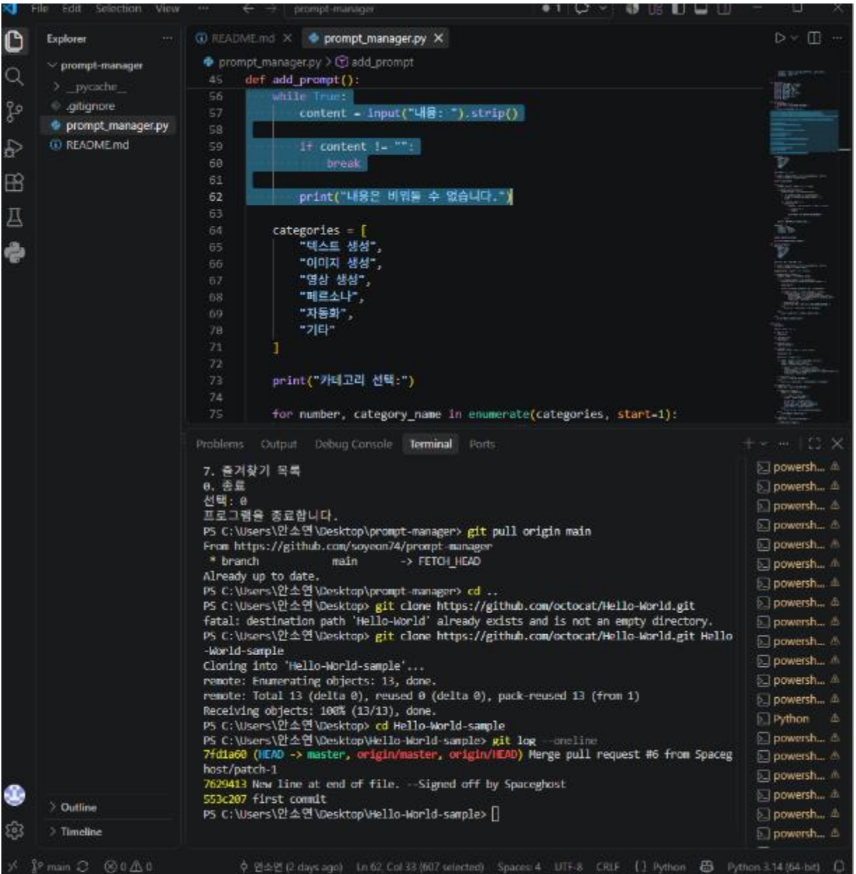
그림 9. git pull 및 공개 저장소 clone-log 확인 화면
