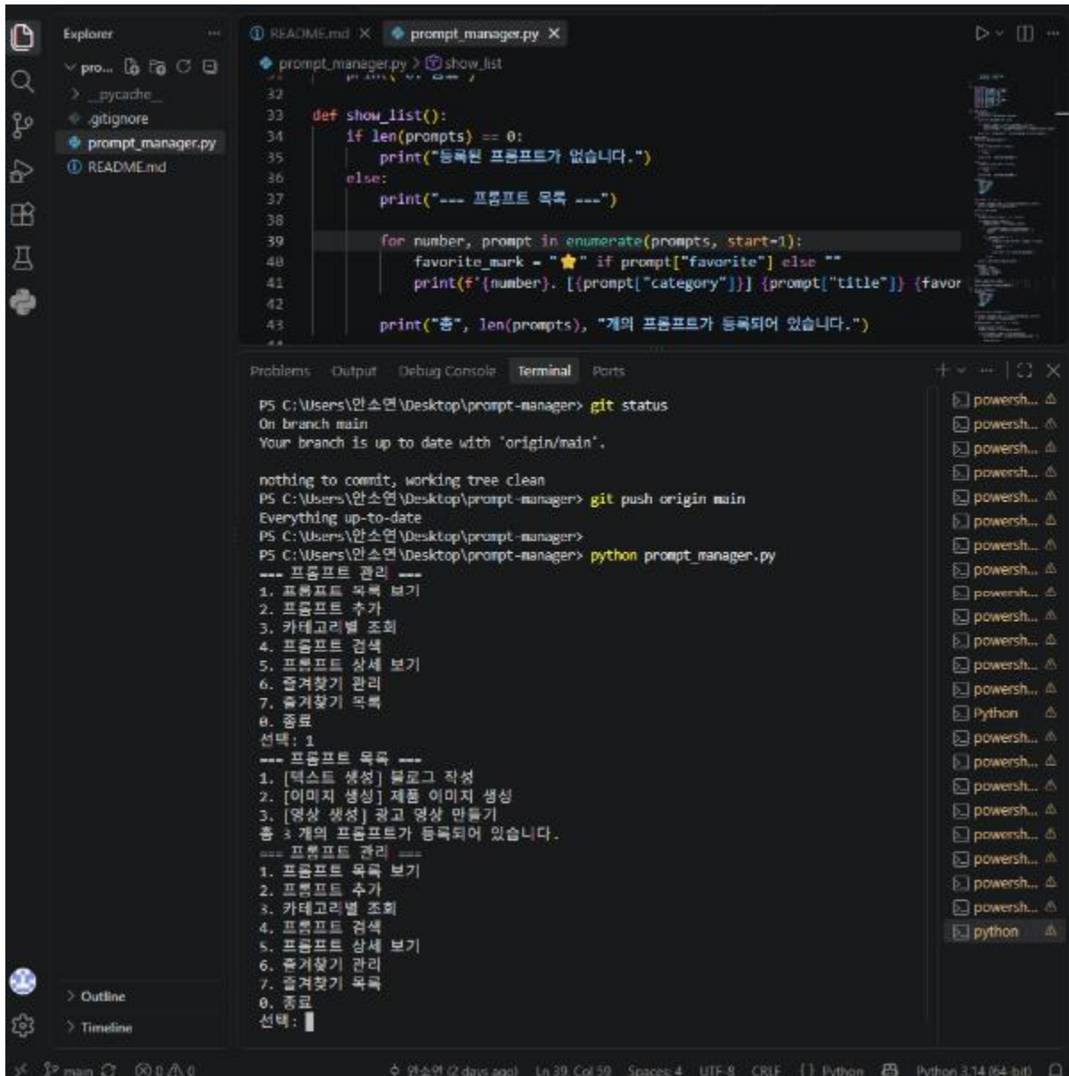
그림 3. 목록 기능 실행 및 기본 데이터 확인
