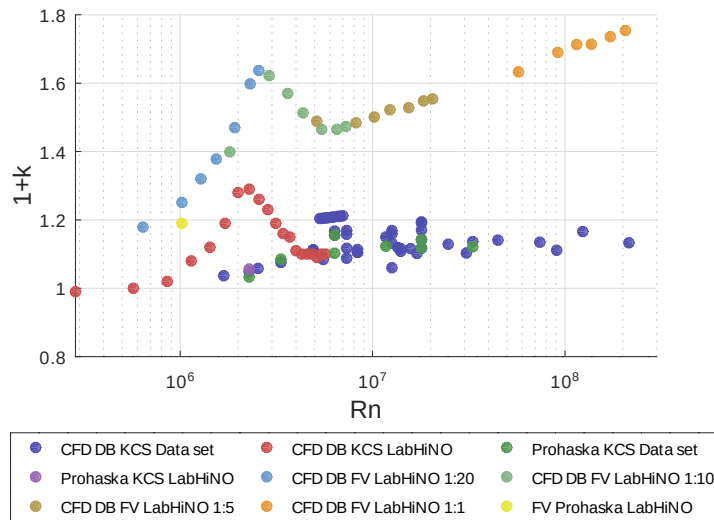
Figura 4.1.24: (1+k) frente a R_n para el KCS y el P1 , en escala logarítmica. Para el KCS se muestran los resultados propios obtenidos en el LabHiNO (CFD DB y Prohaska EFD, escala 1:79) junto con el conjunto de datos recopilado por Terziev et al. [2020] (CFD DB y Prohaska, otras escalas y laboratorios). Para el P1 se muestran únicamente resultados propios: CFD DB en las escalas 1:20, 1:10, 1:5 y 1:1, y el valor experimental obtenido por Prohaska en el LabHiNO (escala 1:20).
