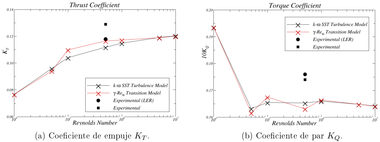
Figura 2.5.1: Coeficientes de empuje y de par frente al número de Reynolds sectional Re_{c,0,7R} . Adaptado de Baltazar et al. [2018].
