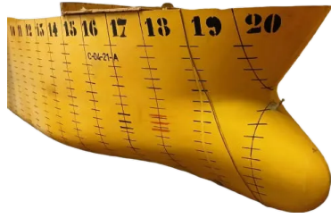
(a) Vista en perspectiva de proa. Se observan las marcas de calado y los estimuladores de turbulencia.
