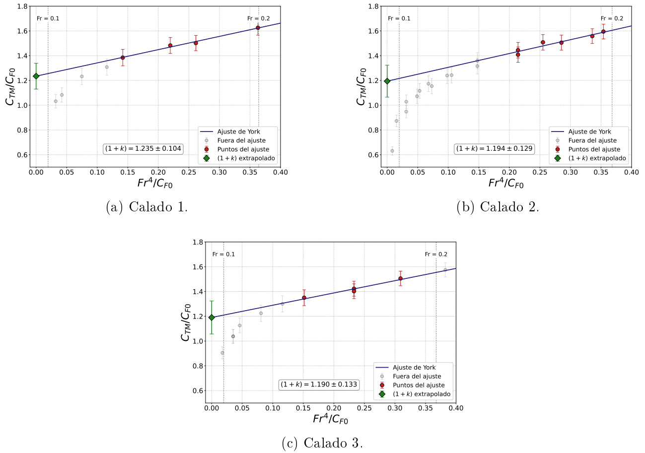
Figura 4.1.4: Ajuste lineal con ponderación mediante el método de York aplicado al P1 para la estimación de (1+k) y su incertidumbre.
