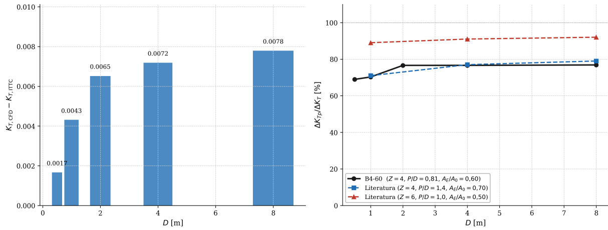
Figura 2.3.3: Izquierda: diferencia K_{T,CFD} - K_{T,ITTC} en función del diámetro. Derecha: fracción del efecto de escala en K_T atribuible a la componente de presión ( \Delta K_{Tp}/\Delta K_T ), comparada con datos de la literatura para otras geometrías.
