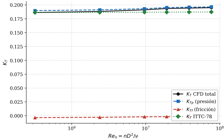
Figura 2.3.1: Coeficientes K_T , K_{Tp} y K_{Tf} en función del número de Reynolds Re_n = nD^2/\nu para el sweep de escala B4-60 a J = 0,5 . Se incluye la predicción del procedimiento ITTC-78 como referencia.
