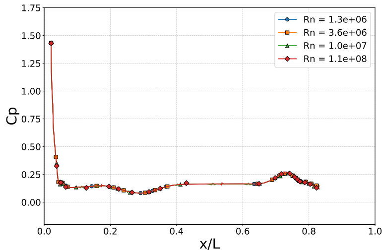
Figura 4.1.35: Distribución de C_P(x/L) sobre el plano z/T = 0,5 .
