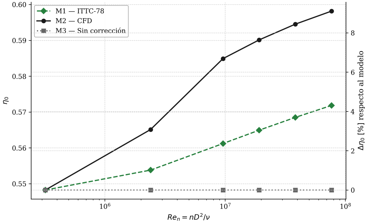
Figura 2.3.5: Eficiencia en aguas abiertas \eta_0 (izquierda) y variación porcentual \Delta\eta_0 respecto al modelo (derecha) en función de Re_n , para los métodos ITTC-78 (M1), CFD SST (M2) y sin corrección (M3). Hélice B4-60, J = 0,5 .
