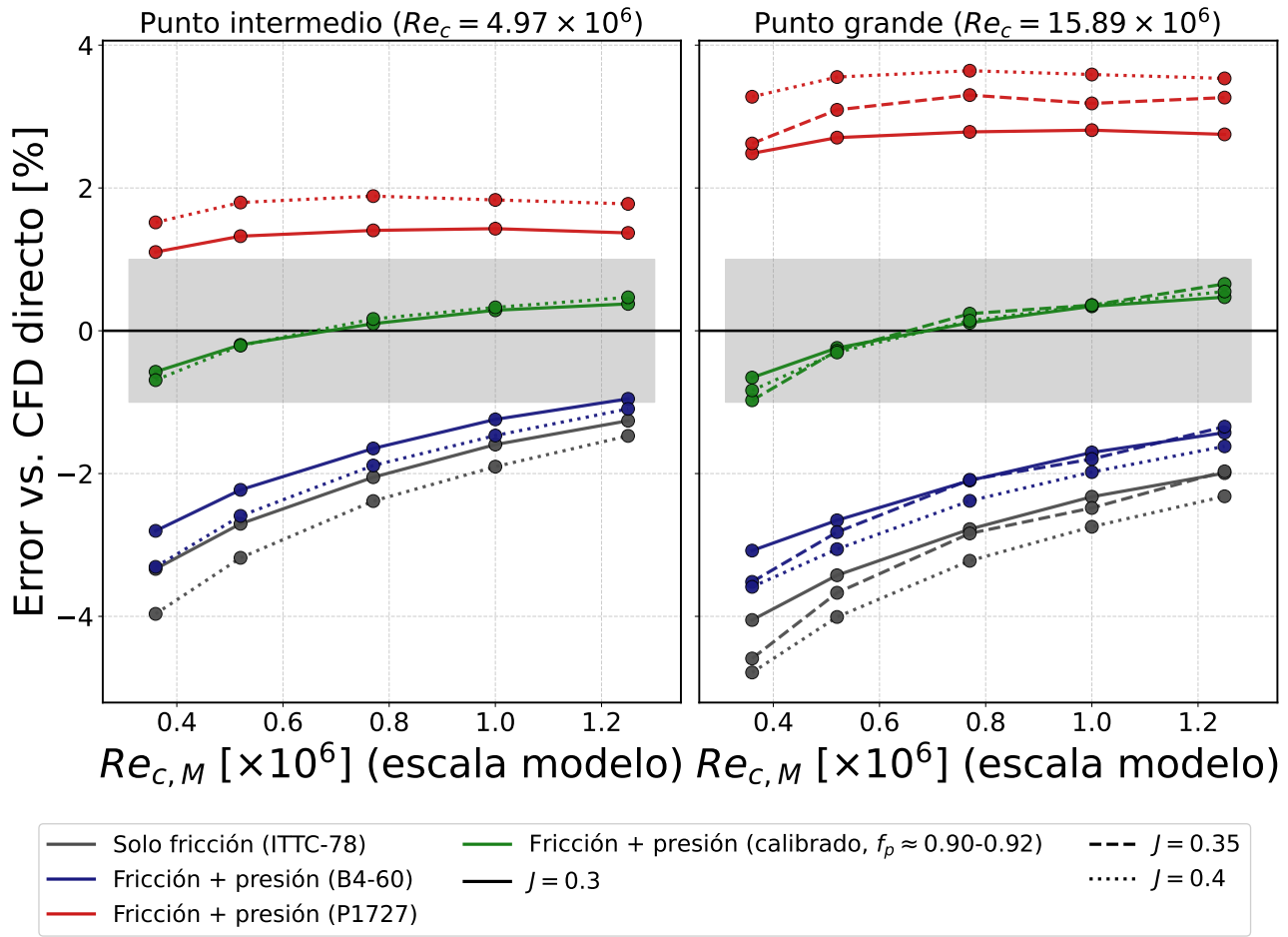
Figura 2.4.2: Error de la extrapolación Fully Turbulent respecto de los dos puntos de validación, para las tres correcciones evaluadas y los tres J calculados.
