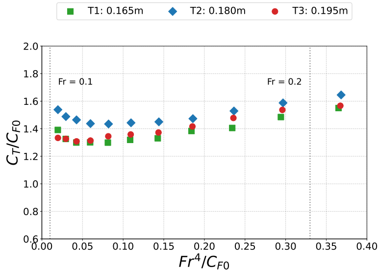
Figura 4.1.11: Diagramas del método de Prohaska para los tres calados del P1 . La desviación respecto de la linealidad teórica se acentúa a bajas números de Froude.
