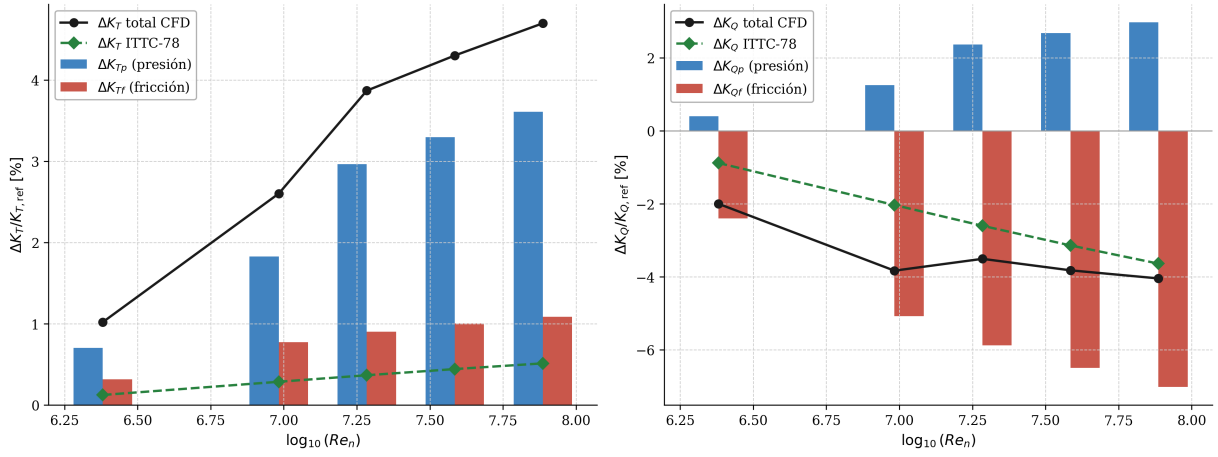
Figura 2.3.2: Variación porcentual de \Delta K_T (izquierda) y \Delta K_Q (derecha) respecto al caso de referencia D = 0,14 m, descompuesta en contribuciones de presión y fricción. Se incluye la predicción del ITTC-78.
