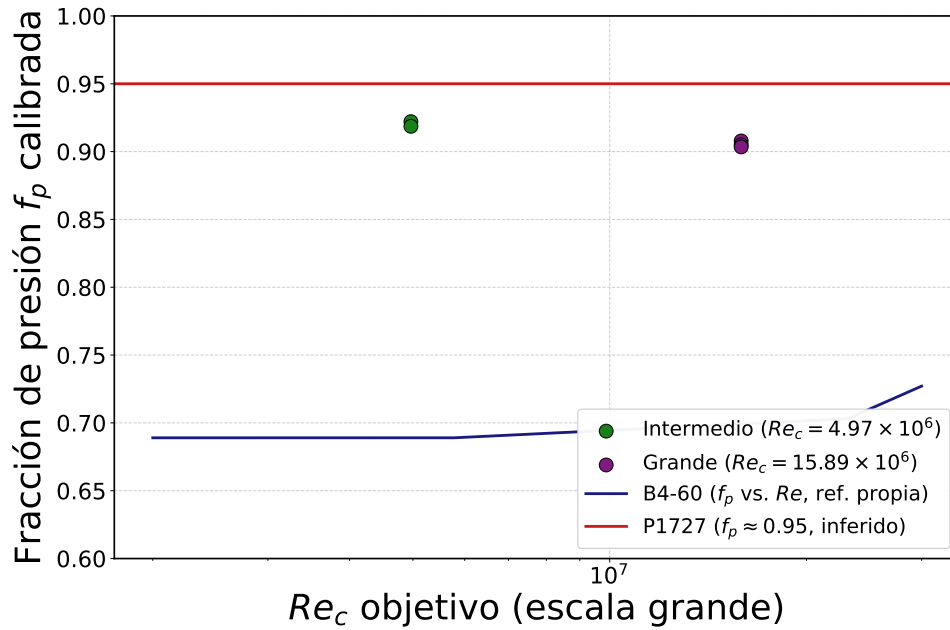
Figura 2.4.1: Fracción de presión calibrada en los dos puntos de escala independientes, comparada con la curva propia de la B4-60 (evaluada en función de Re ) y con el valor inferido del P1727.
