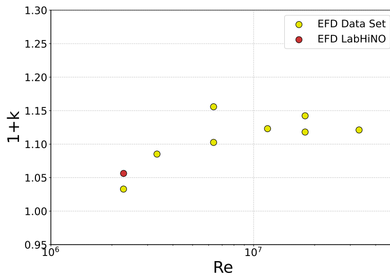
Figura 4.1.8: Comparación del factor de forma ( 1+k ) del KCS obtenido en el LabHiNO (punto rojo) con resultados experimentales históricos del KCS compilados de literatura internacional en Terziev et al. [2020] (puntos amarillos), en función del número de Reynolds.
