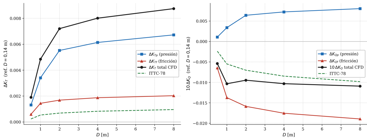
Figura 2.3.4: Variación de \Delta K_T (izquierda) y 10\Delta K_Q (derecha) en función del diámetro, con descomposición en componentes de presión y fricción. Se incluye la predicción del ITTC-78.
