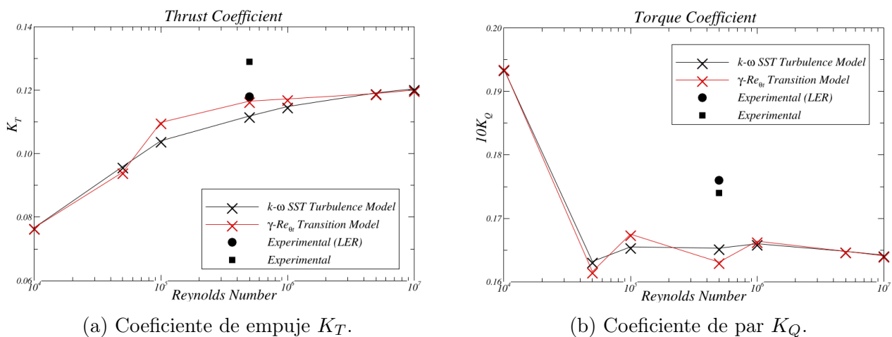
Figura 2.5.1: Coeficientes de empuje y de par frente al número de Reynolds seccional Re_{c,0.7R} . Adaptado de Baltazar et al. [2018].
