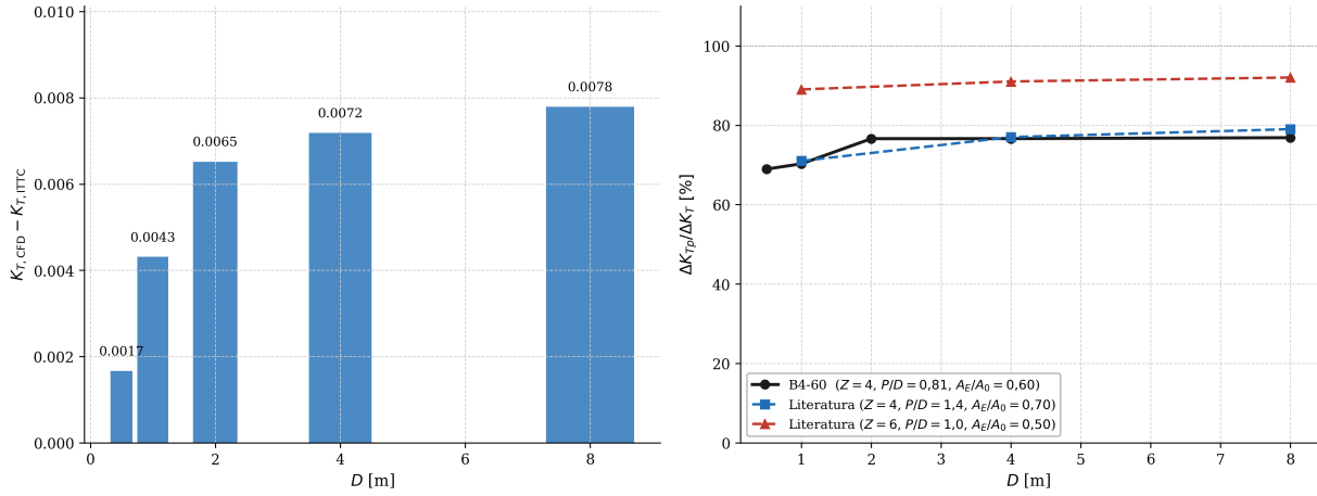
Figura 5.3.3: Izquierda: diferencia K_{T,CFD} - K_{T,ITTC} en función del diámetro. Derecha: fracción del efecto de escala en K_T atribuible a la componente de presión ( \Delta K_{Tp}/\Delta K_T ), comparada con datos de la literatura para otras geometrías.
