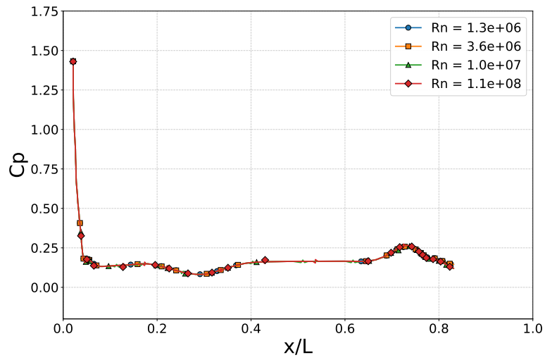
Figura 4.1.34: Distribución de C_P(x/L) sobre el plano z/T = 0,5 .
