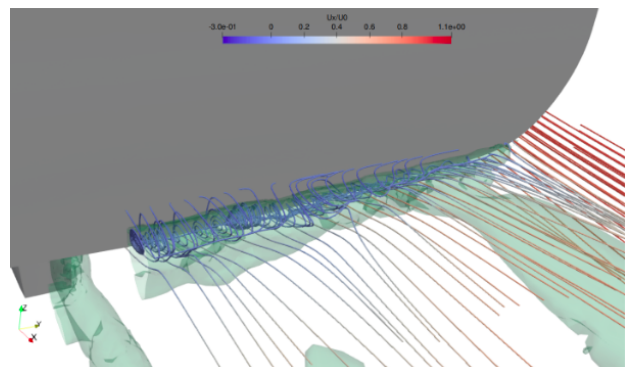
(d) Escala buque, Fr = 0.36
