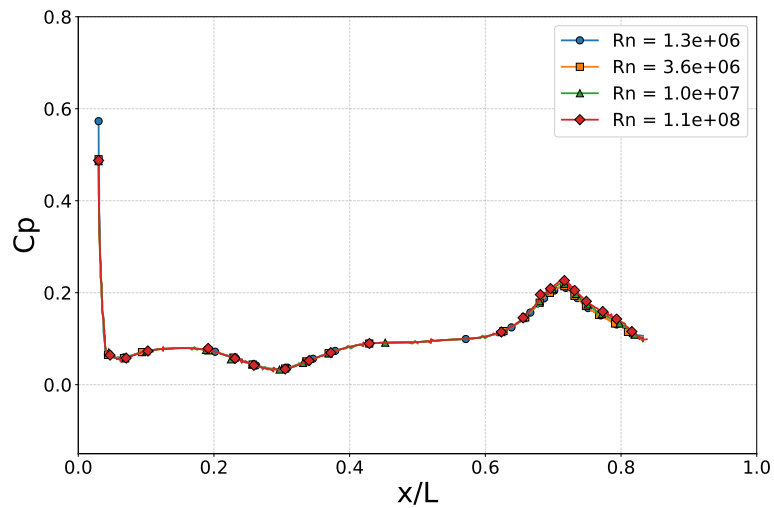
Figura 4.1.35: Distribución de C_P(x/L) sobre el plano z/T = 0,75 .
