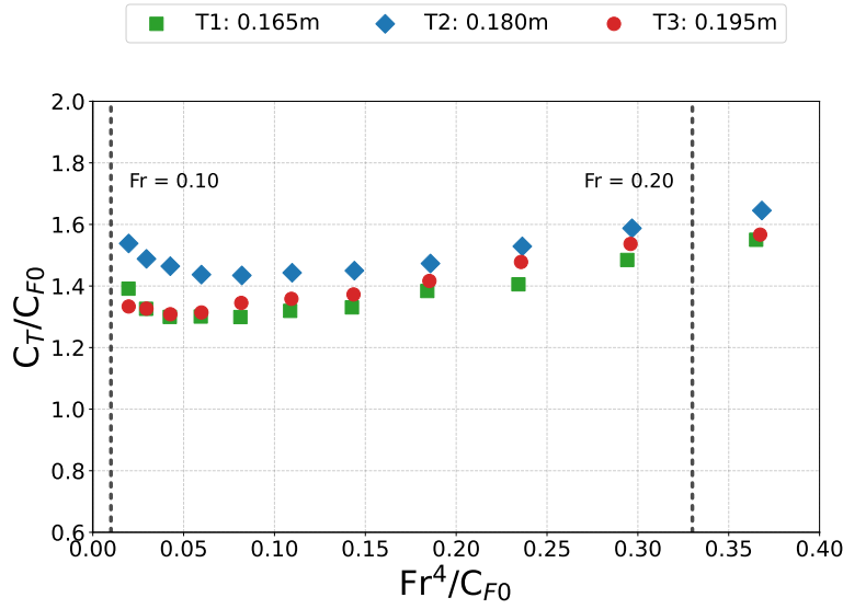
Figura 4.1.15: Diagramas del método de Prohaska para los tres calados del P1 . La desviación respecto de la linealidad teórica se acentúa a bajos números de Froude. Las líneas verticales punteadas indican Fr = 0.10 y Fr = 0.20 para el P1 .
