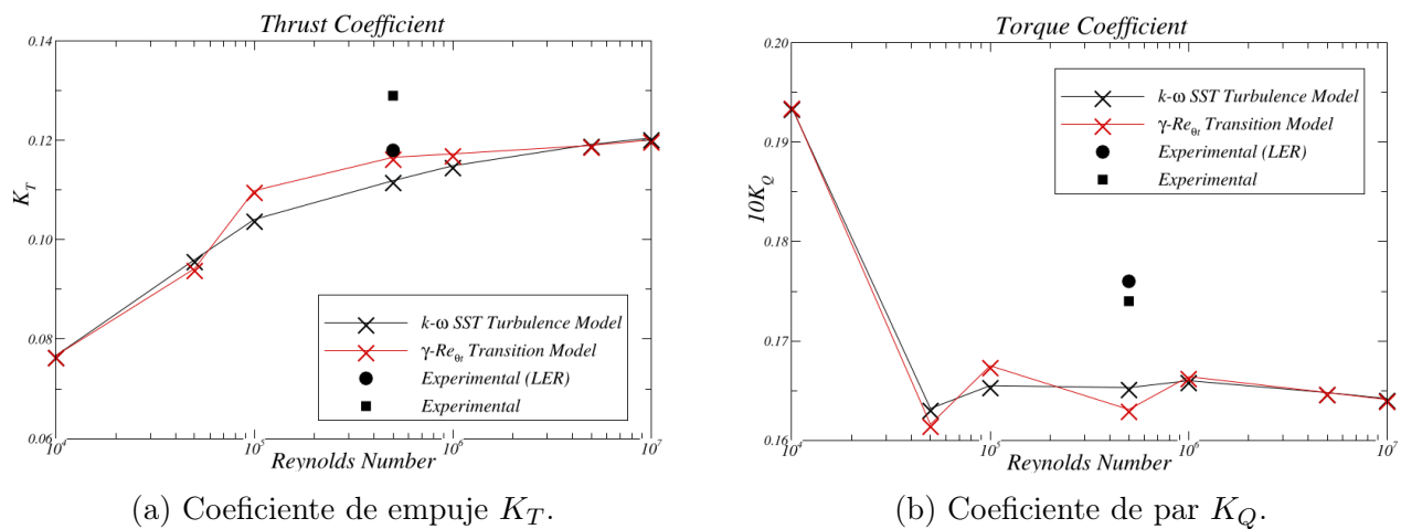
Figura 2.5.1: Coeficientes de empuje y de par frente al número de Reynolds sectional Re_{c,0.7R} . Adaptado de Baltazar et al. [2018].
