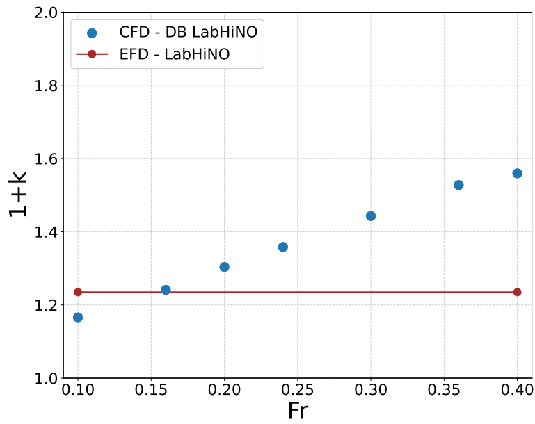
Figura 4.1.29: Comparación entre el valor de (1+k) adoptado por Prohaska (línea horizontal roja) y los valores obtenidos mediante el método de doble cuerpo en función de Fr (puntos azules) para el P1 , Calado 1.
