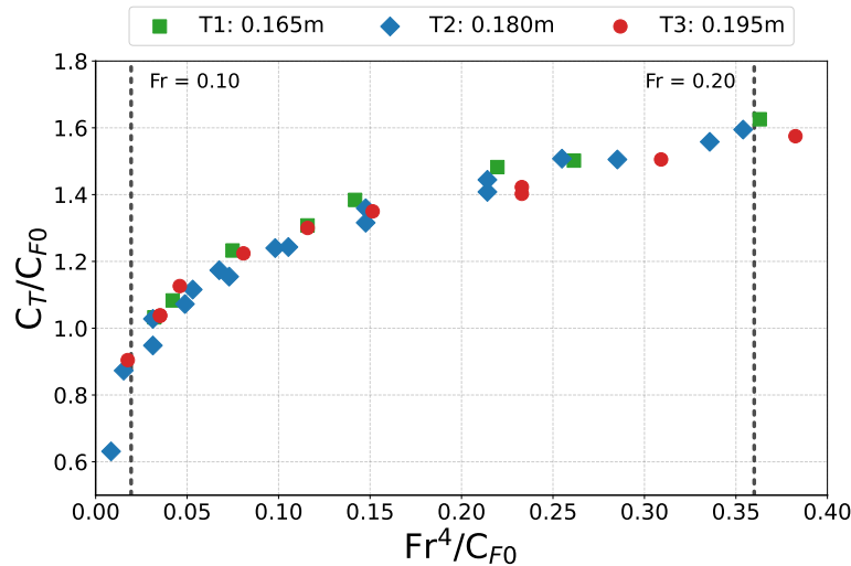
Figura 4.1.4: Diagramas del método de Prohaska para los tres calados del P1 . La desviación respecto de la linealidad teórica se acentúa a bajos números de Froude.
