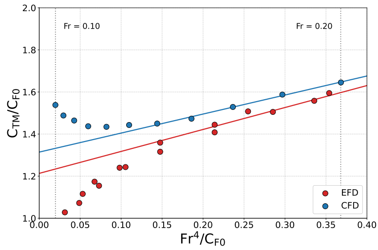
Figura 4.1.24: Diagrama de Prohaska del P1 comparando EFD y CFD. Calado 2.
