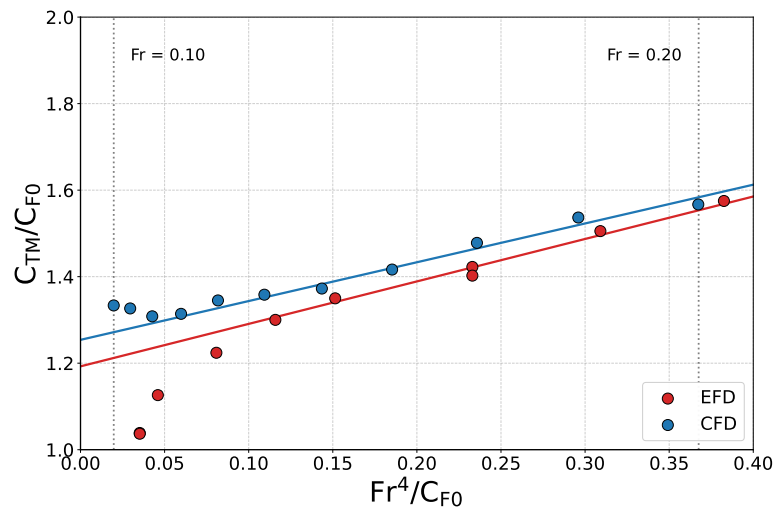
Figura 4.1.25: Diagrama de Prohaska del P1 comparando EFD y CFD. Calado 3.
