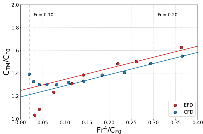
Figura 4.1.23: Diagrama de Prohaska del P1 comparando EFD y CFD. Calado 1.
