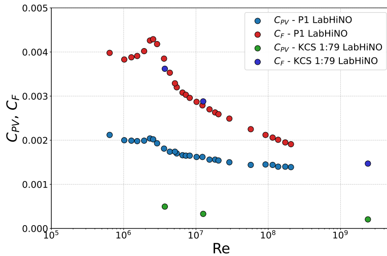
Figura 4.1.37: C_{PV} y C_F obtenidos mediante CFD en doble cuerpo para el P1 y para el KCS 1:79 (LabHiNO).
