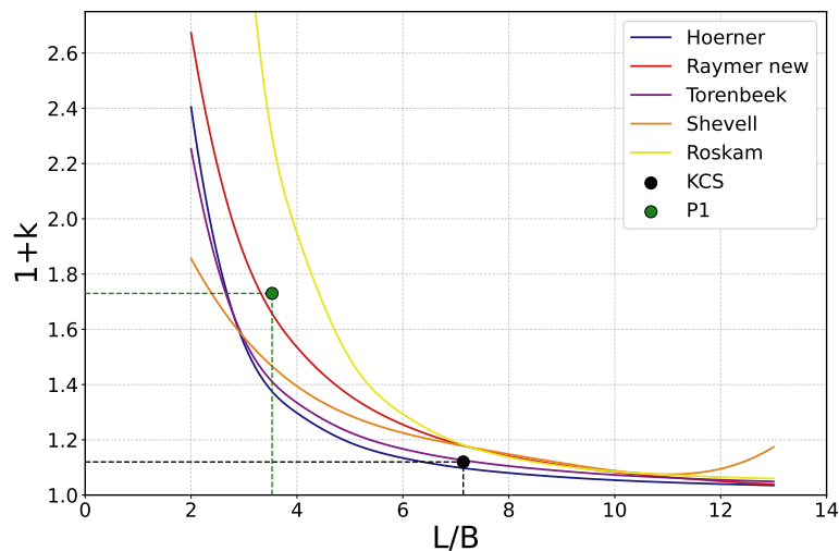
Figura 4.6.3: Factores de forma para cuerpos de revolución en función de la razón de esbeltez l/d y comparación con valores CFD DB para el P1 y el KCS. Datos de [Hoerner, 1965, Raymer, 2019, Torenbeek, 2010, Roskam, 1987, Shevell, 1989, Terziev et al., 2020].
