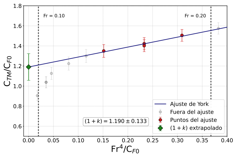
Figura 4.1.6: Ajuste lineal con ponderación mediante el método de York aplicado al P1 para la estimación de (1+k) y su incertidumbre.
