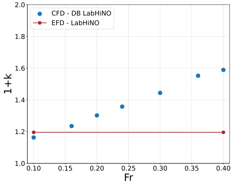
Figura 4.1.30: Comparación entre el valor de (1+k) adoptado por Prohaska (línea horizontal roja) y los valores obtenidos mediante el método de doble cuerpo en función de Fr (puntos azules) para el P1 , Calado 2.
