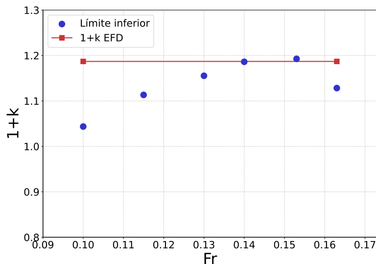
Figura 4.1.5: Variación del factor de forma (1+k) al modificar el límite inferior del rango de Froude (puntos azules), manteniendo el superior en Fr = 0.20 . La línea roja indica el valor de (1+k) adoptado mediante el método de Prohaska en el rango 0.15 < Fr < 0.20 . Calado 3. Comportamiento análogo en otros calados.
