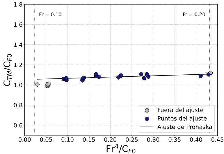
Figura 4.1.7: Diagrama de Prohaska para el modelo KCS. Se grafica C_{TM}/C_{F0} frente a Fr^4/C_{F0} , donde C_{F0} es el coeficiente de fricción de placa plana al Re del modelo según la línea ITTC-57. La línea continua representa el ajuste por mínimos cuadrados, cuya extrapolación al origen permite obtener el valor de 1 + k .
