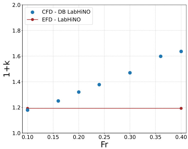
Figura 4.1.31: Comparación entre el valor de (1+k) adoptado por Prohaska (línea horizontal roja) y los valores obtenidos mediante el método de doble cuerpo en función de Fr (puntos azules) para el P1 , Calado 3.
