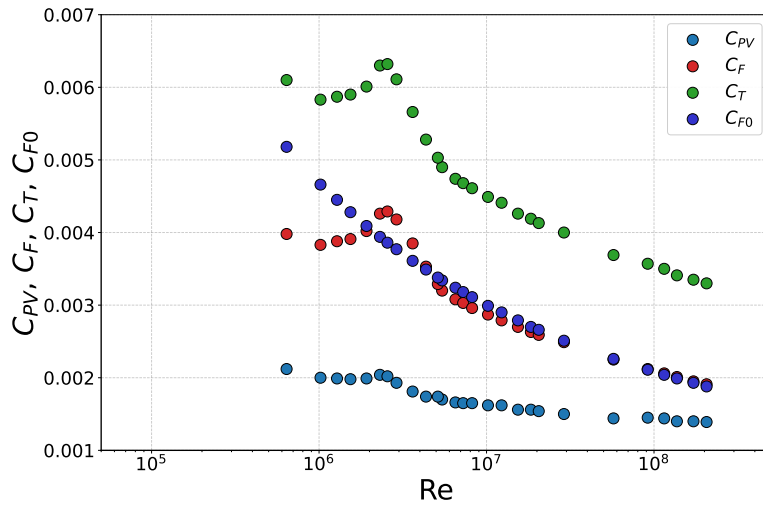
Figura 4.1.36: Coeficientes C_T , C_{PV} y C_F obtenidos mediante CFD en configuración de doble cuerpo, junto con la línea ITTC-57 ( C_{F0} ), en función de Re para el P1 .
