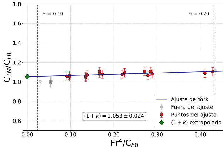
Figura 4.1.8: Ajuste lineal con ponderación mediante el método de York aplicado al KCS para la estimación de (1+k) y su incertidumbre.
