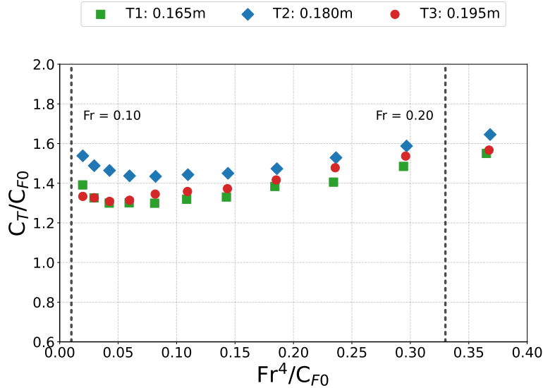
Figura 4.1.15: Diagramas del método de Prohaska para los tres calados del P1 . La desviación respecto de la linealidad teórica se acentúa a bajos números de Froude.
