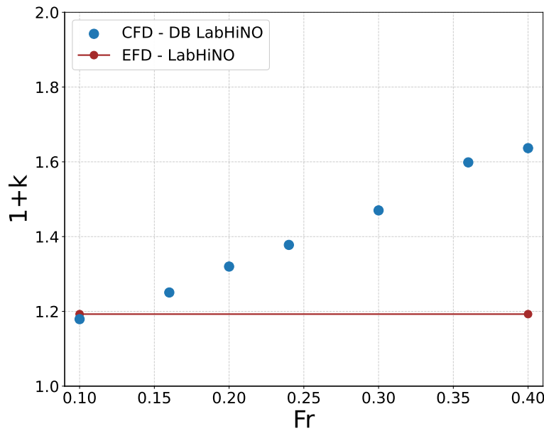
Figura 4.1.31: Comparación entre el valor de (1+k) adoptado por Prohaska (línea horizontal roja) y los valores obtenidos mediante el método de doble cuerpo (DB) en función de Fr (puntos azules) para el P1 , Calado 3.
