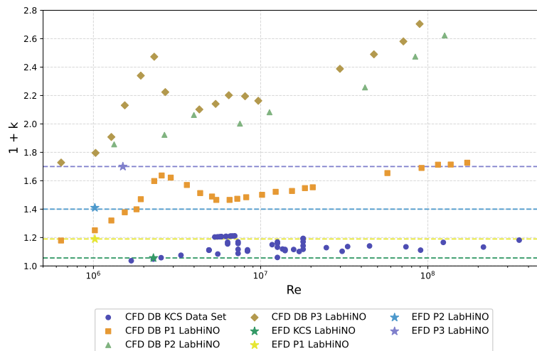
Figura 4.1.34: Evolución de (1+k) con el número de Reynolds para el KCS y los tres pesqueros analizados.
