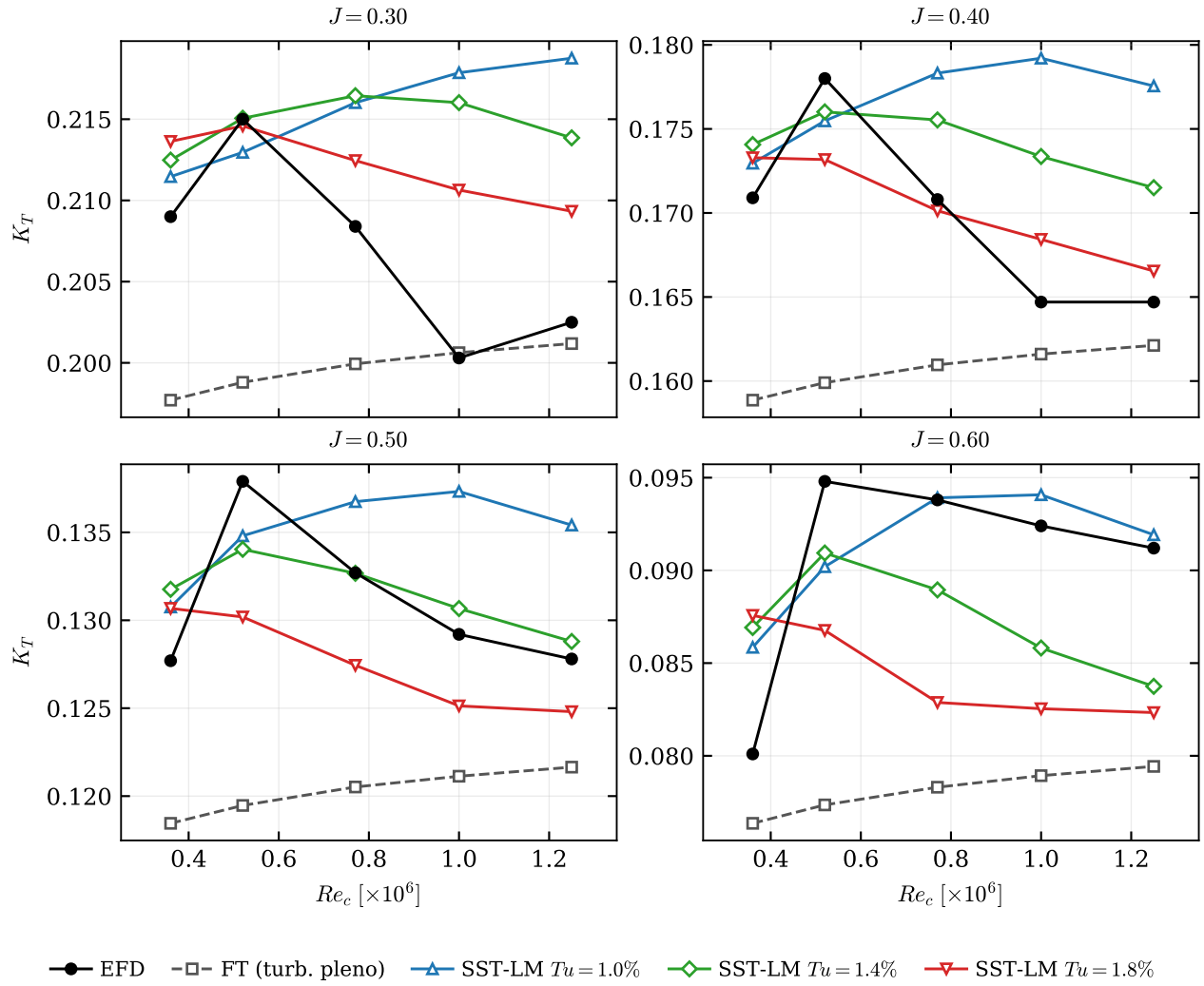
Figura 5.4.3: Coeficiente de empuje K_T en función de Re_c para cuatro valores de J , calculado con StarCCM+ . Configuraciones análogas a las de la Figura 5.4.1.
