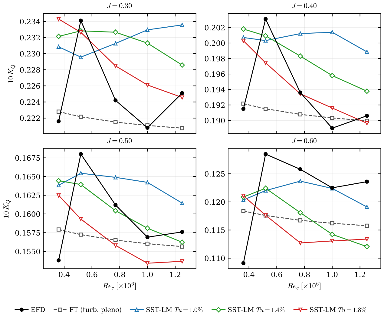
Figura 5.4.4: Coeficiente de par 10K_Q en función de Re_c para cuatro valores de J , calculado con StarCCM+ . Configuraciones análogas a las de la Figura 5.4.1.
