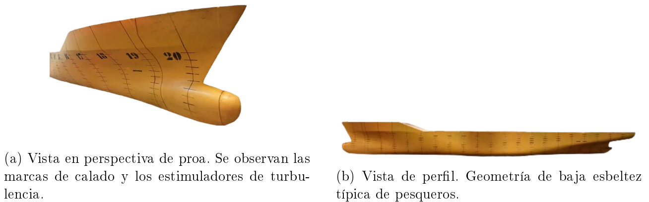
Figura 3.2.4: Modelo físico del KCS (Escala 1:79) preparado para ensayos en el LabHiNO.
