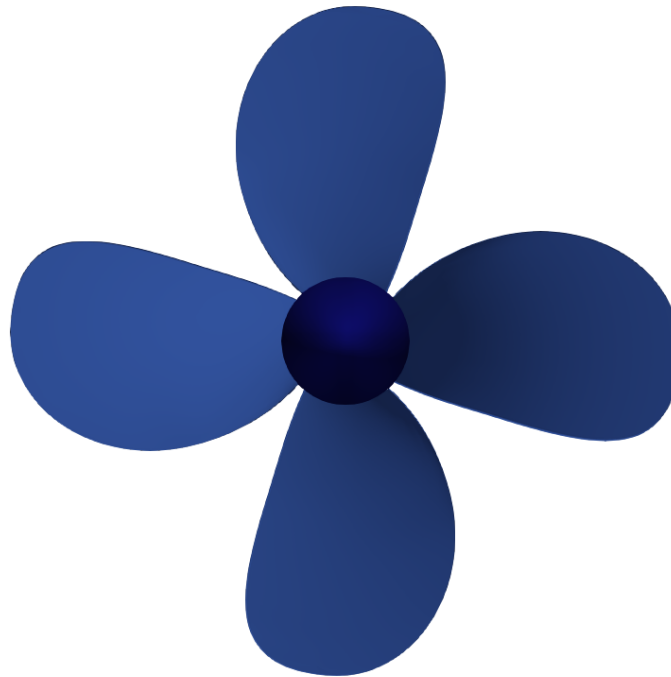
Figura 3.2.5: Geometría de la hélice de referencia Wageningen B4-60.
