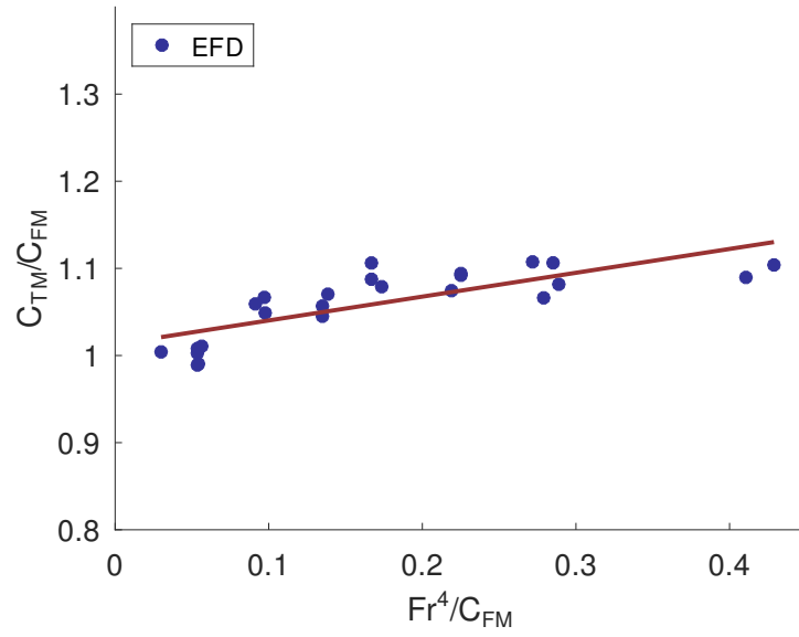
Figura 4.1.4: Determinación experimental del factor de forma (1 + k) para el modelo KCS mediante el método de Prohaska.
