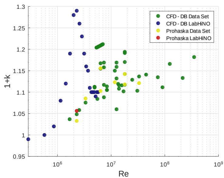
Figura 4.1.6: Comparación del factor de forma (1 + k) del KCS obtenido en el LabHiNO con resultados internacionales.
