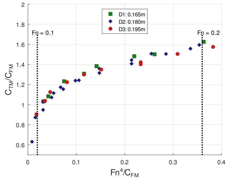
Figura 4.1.1: Diagramas del método de Prohaska para los tres calados del pesquero TPA. La desviación respecto de la linealidad teórica se acentúa a bajos números de Froude.
