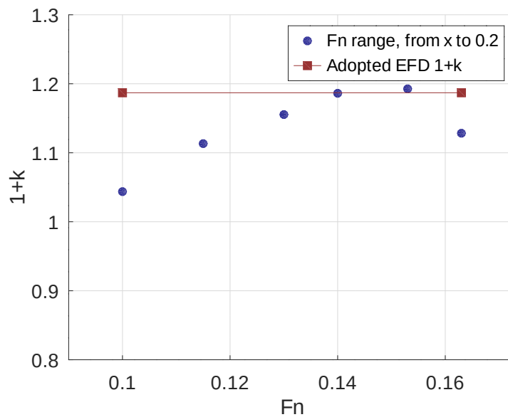
Figura 4.1.2: Variación del factor de forma experimental ( 1+k ) para el pesquero TPA en función del rango de Froude utilizado en el ajuste de Prohaska.
