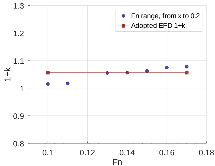
Figura 4.1.5: Variación del factor de forma (1 + k) para el modelo KCS en función del rango de Froude considerado en el ajuste de Prohaska.
