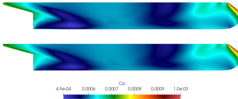
Figura 4.1.34: C_P para F_n = 0,2 , vista lateral. Arriba: escala 1:20. Abajo: escala 1:1.
