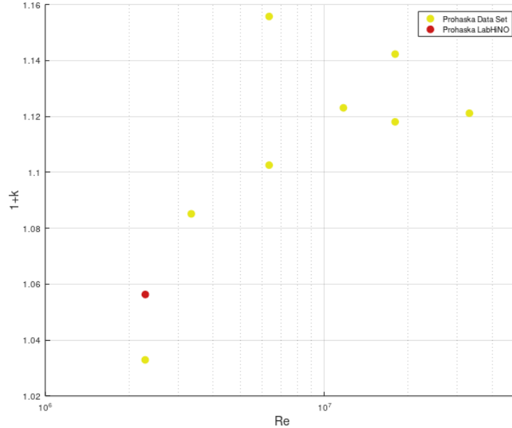
Figura 4.1.7: Comparación del factor de forma (1+k) del KCS obtenido en el LabHiNO (punto rojo) con resultados de distintos laboratorios internacionales recopilados por Terziev et al. [2020] (puntos amarillos), en función del número de Reynolds.
