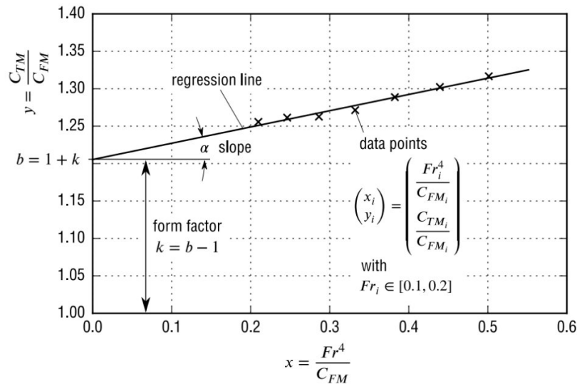
Figura 2.1.3: Método de Prohaska para determinar el factor de forma k . La ordenada al origen de la regresión lineal sobre el rango Fr \in [0,1; 0,2] da (1 + k) . Adaptado de ?.
