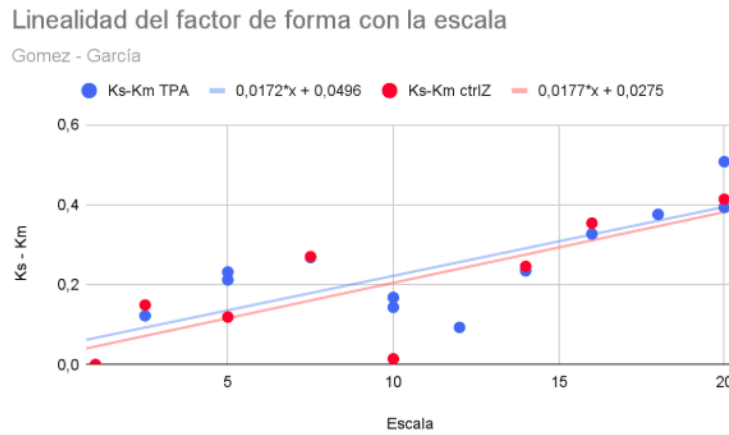
Figura 4.1.26: Linealidad del factor de forma con la escala para el P1 , siguiendo el método de Garcia-Gómez [2000].
