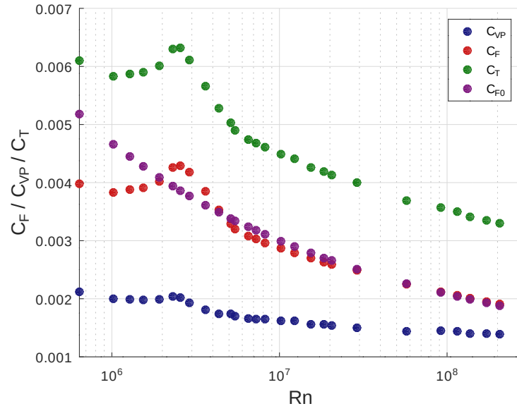
Figura 4.1.27: Coeficientes C_T , C_{PV} y C_F obtenidos mediante CFD en configuración de doble cuerpo, junto con la línea ITTC-57 ( C_{F0} ), en función de R_n para el P1 .
