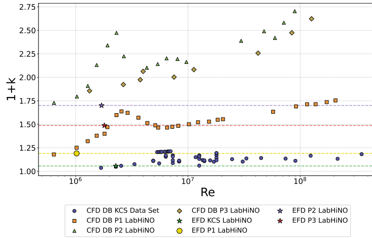
Figura 4.1.23: Evolución de (1+k) con el número de Reynolds para el KCS y los tres pesqueros analizados.
