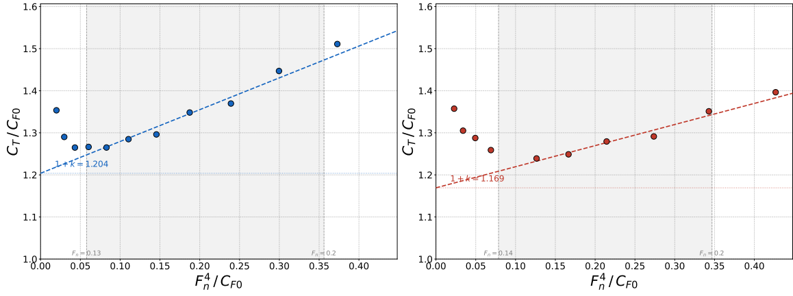
Figura 4.2.2: Diagrama de Prohaska comparando modelos con y sin bulbo ( T = 0,165 m).
