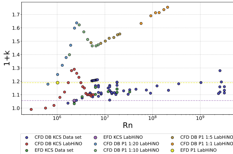
Figura 4.1.22: (1+k) frente a Re para el KCS y el P1 , en escala logarítmica. Para el KCS se muestran los resultados propios obtenidos en el LabHiNO (CFD DB y Prohaska EFD, escala 1:79) junto con el conjunto de datos recopilado por Terziev et al. [2020] (CFD DB y Prohaska, otras escalas y laboratorios). Para el P1 se muestran únicamente resultados propios: CFD DB en las escalas 1:20, 1:10, 1:5 y 1:1, y el valor experimental obtenido por Prohaska en el LabHiNO (escala 1:20).
