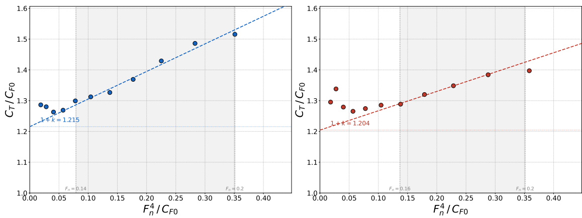
Figura 4.2.3: Diagrama de Prohaska comparando modelos con y sin bulbo ( T = 0,195 m).
