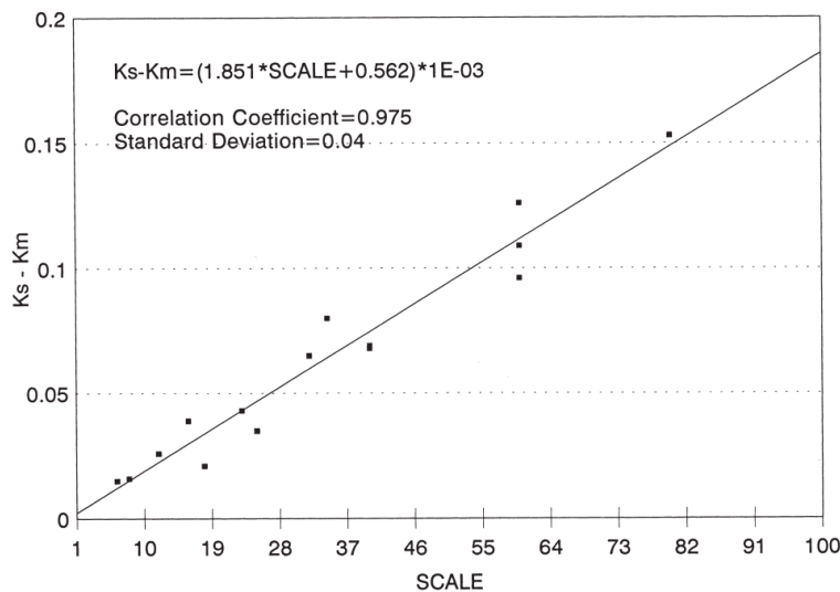
Figura 2.1.1: Efecto de escala del factor de forma, K_S - K_M , en función de la razón de escala \lambda para quince modelos de cuatro familias de geosims, con la recta de regresión de García-Gómez [2000] .
