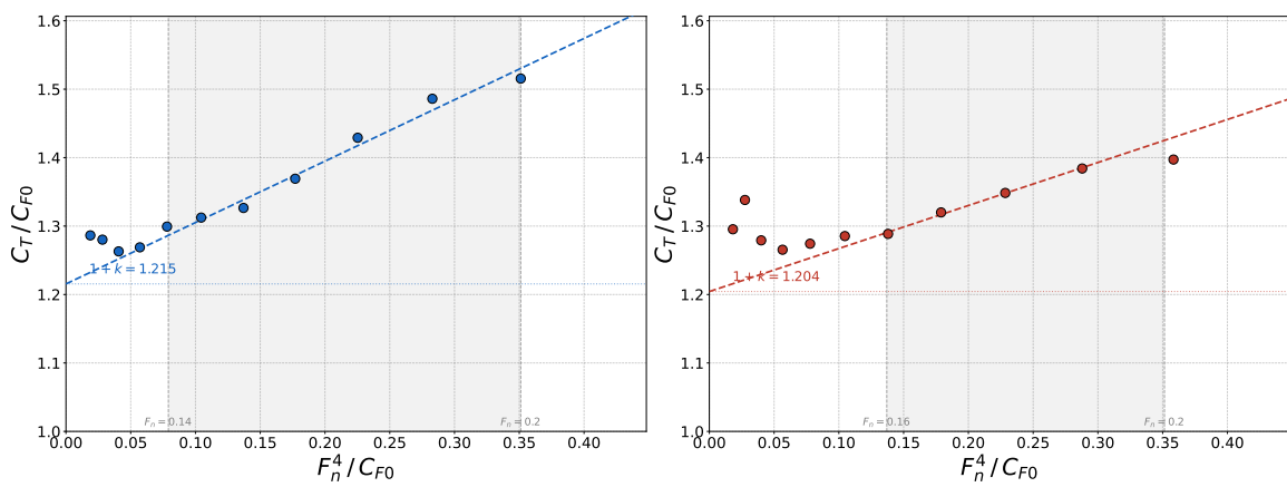
Figura 4.2.3: Diagrama de Prohaska comparando modelos con y sin bulbo ( T = 0,195 m).
