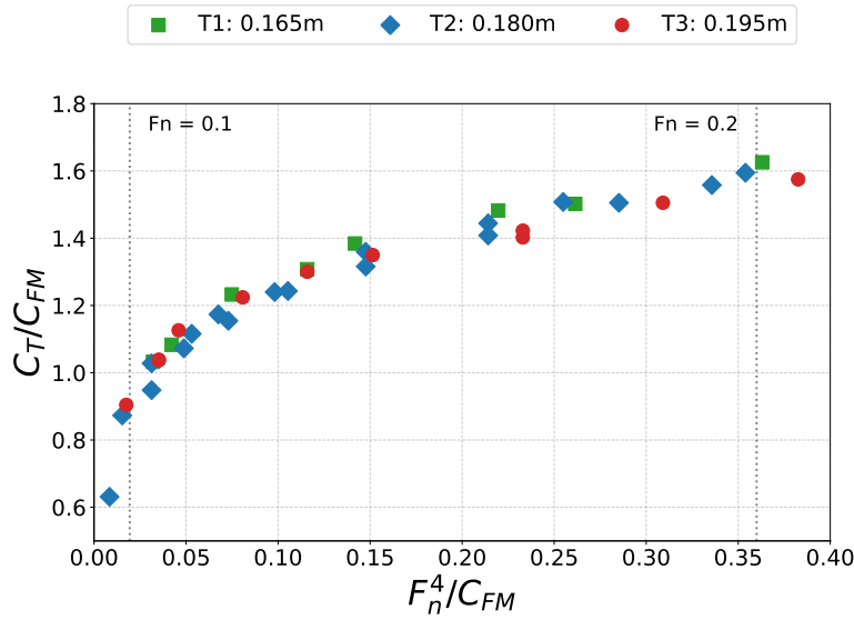
Figura 4.1.2: Diagramas del método de Prohaska para los tres calados del P1 . La desviación respecto de la linealidad teórica se acentúa a bajos números de Froude.
