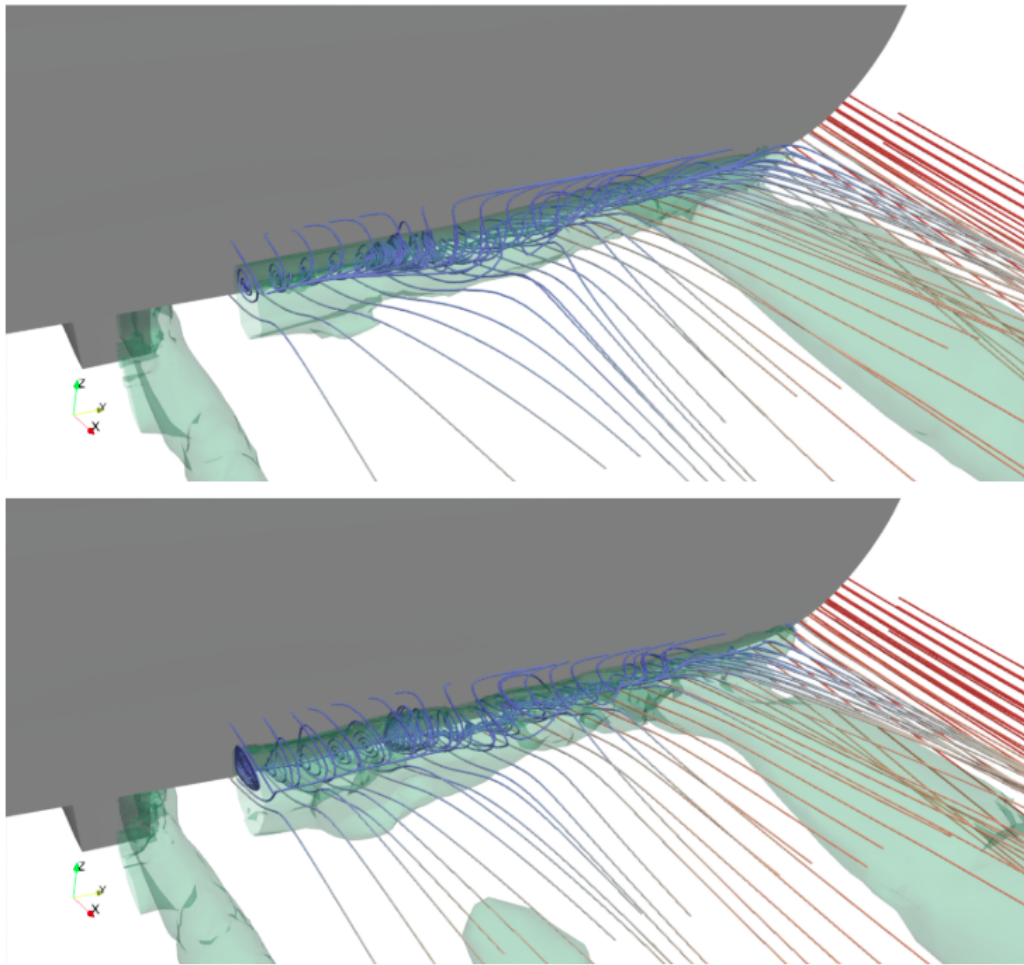
Figura 4.1.39: Iso-superficies de Q -criterion ( Q=10 ) mostrando las estructuras vorticosas presentes en la popa, a escala modelo, 1:20 (arriba, \log(Re) \approx 6 ) y escala buque, 1:1 (abajo, \log(Re) \approx 8 ), a Fr = 0.2 .
