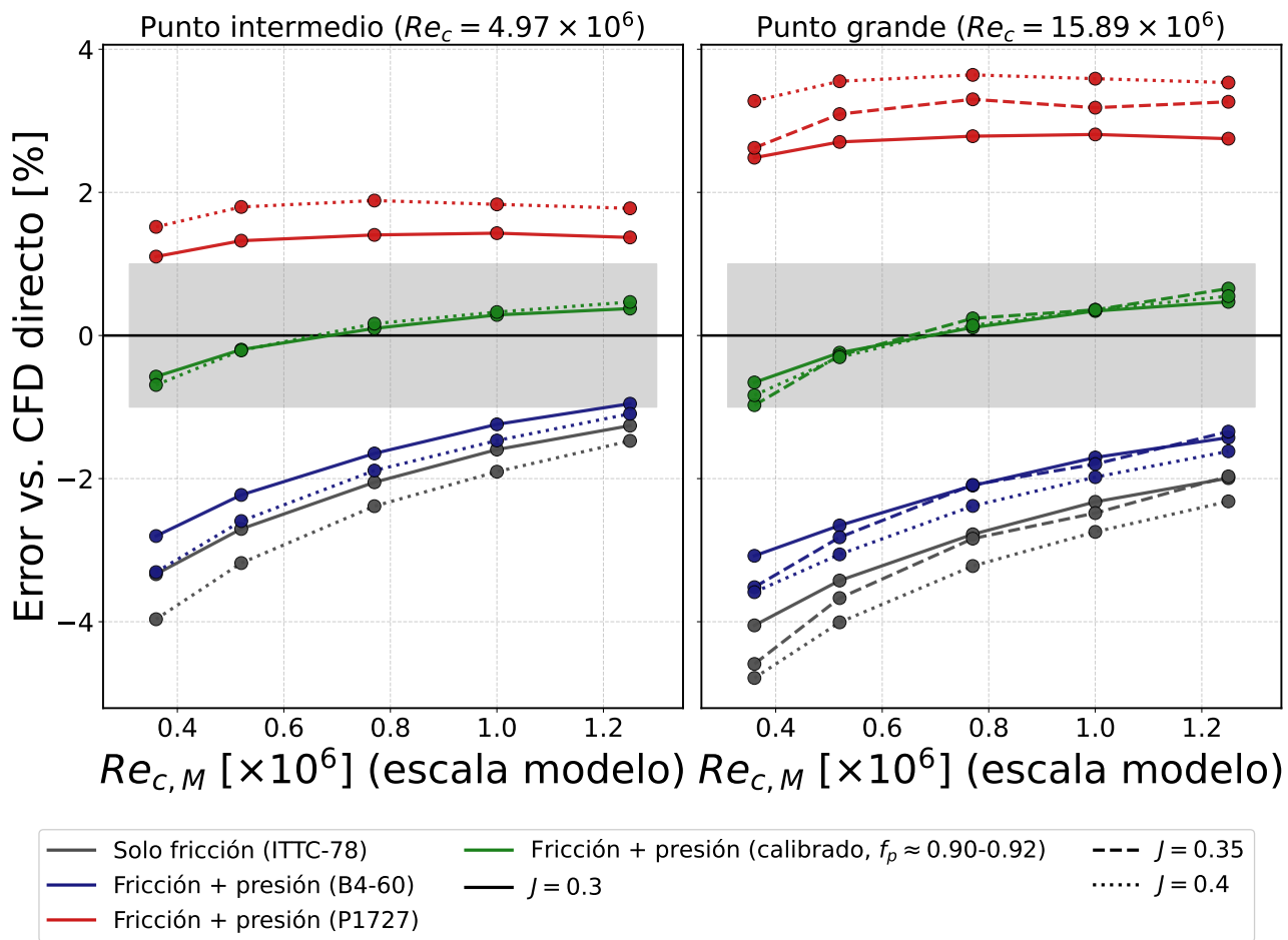
Figura 5.4.2: Error de la extrapolación Fully Turbulent respecto de los dos puntos de validación, para las tres correcciones evaluadas y los tres J calculados.
